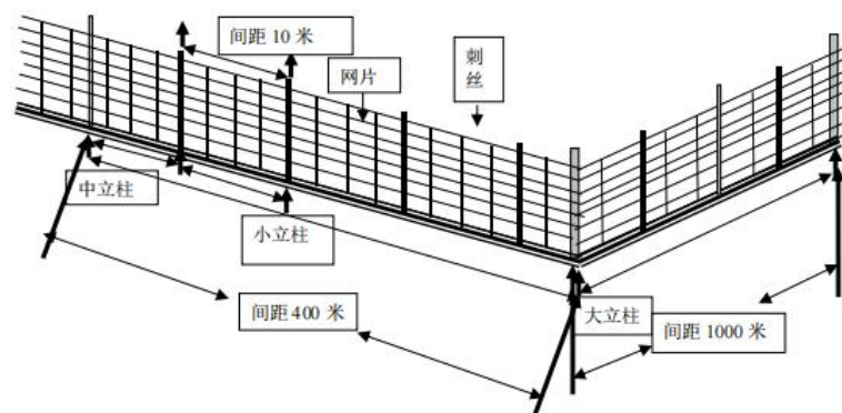
角铁立柱式网围栏装示意图
