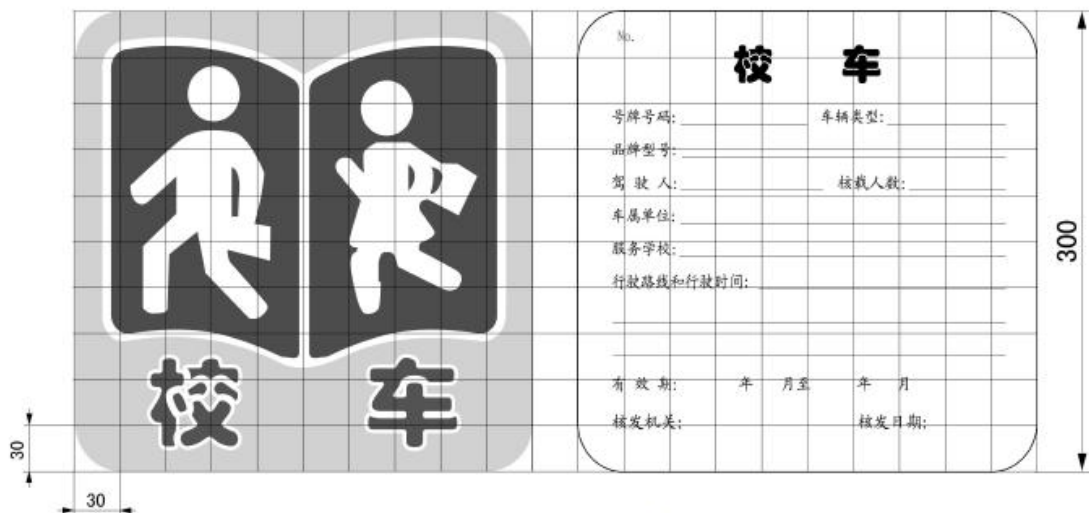
图5 校车标牌尺寸
