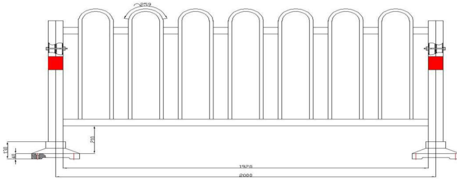
标准段立面图
