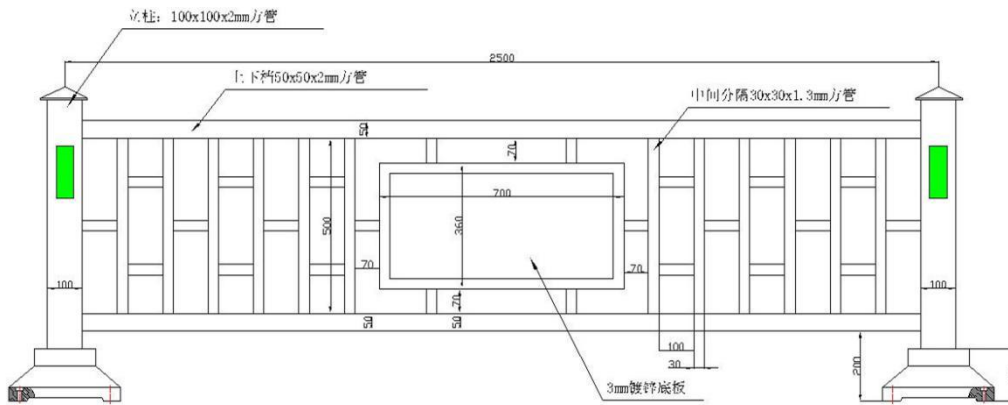
标准段立面图
