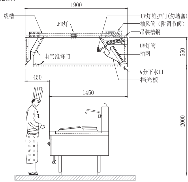
截面示意图
