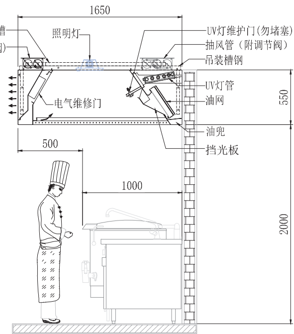
截面示意图
