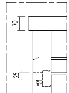
Detail-A SC=1:3
