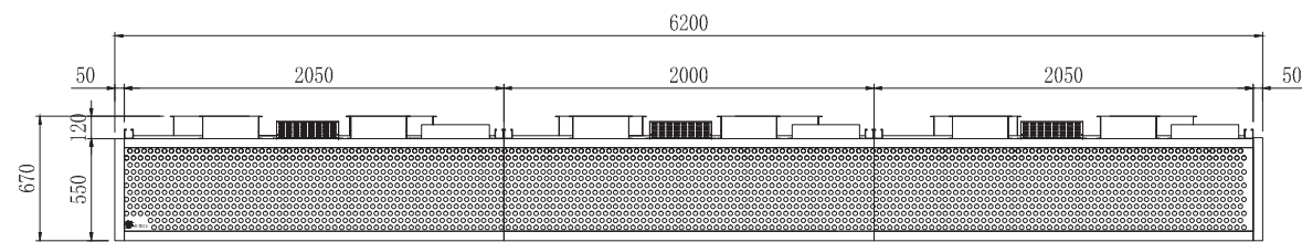
正视图
