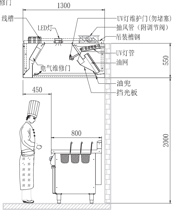
截面示意图
