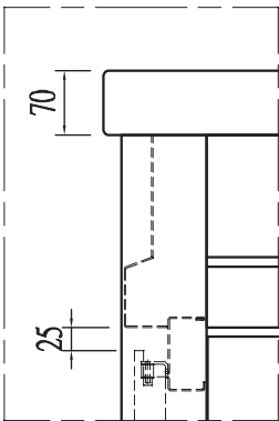
Detail-A SC=1:3
