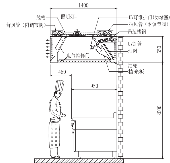
截面示图
