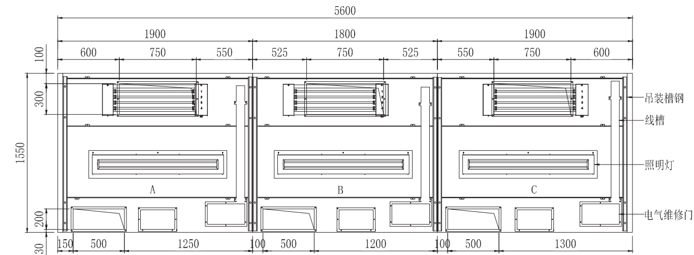
俯视图
