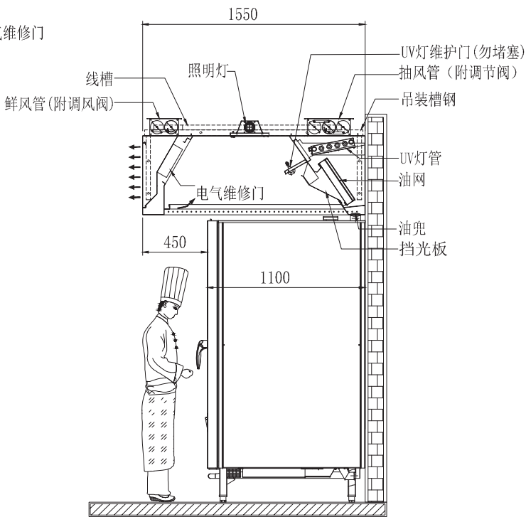
截面示意图
