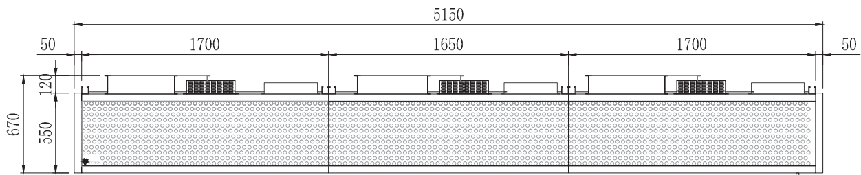
正视图
