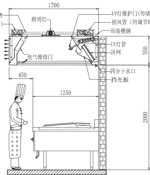
截面示意图
