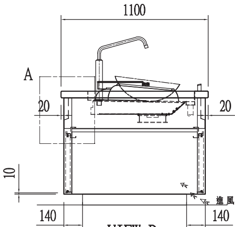
VIEW-D
