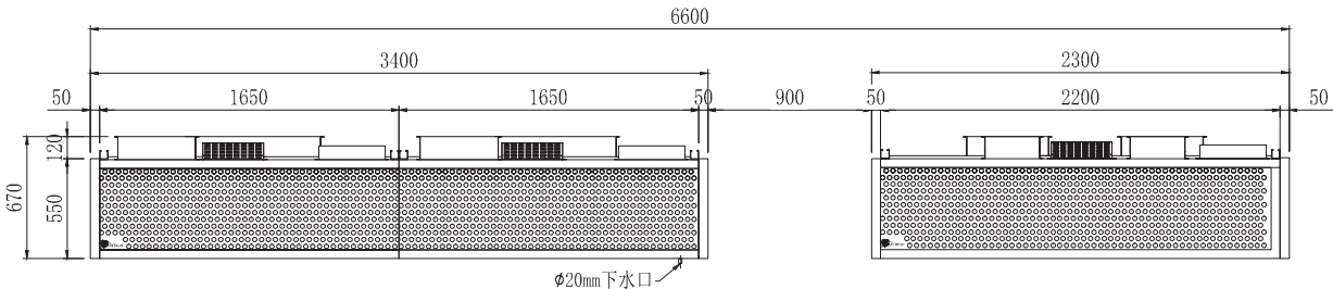
正视图
