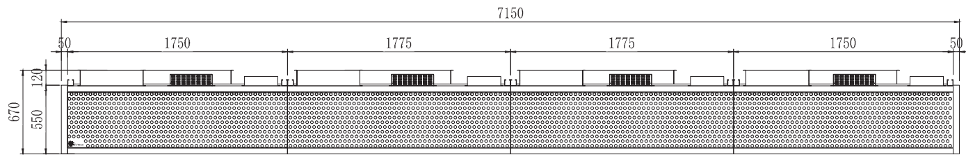
正视图
