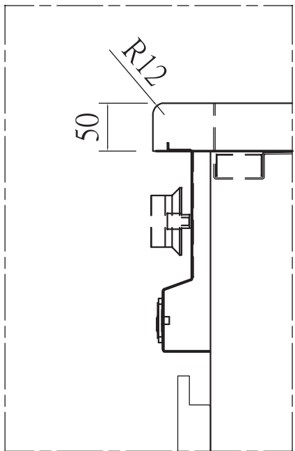
Deatil-A
