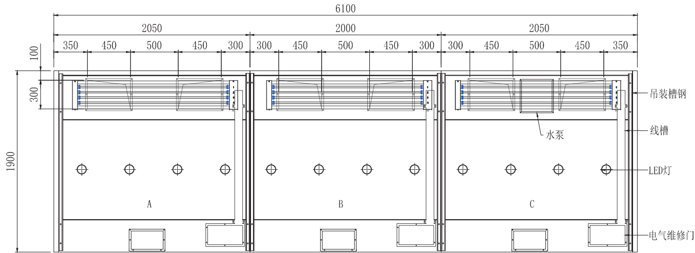
俯视图
