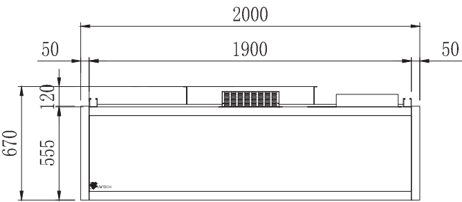
正视图
