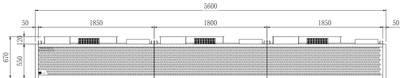
正视图
