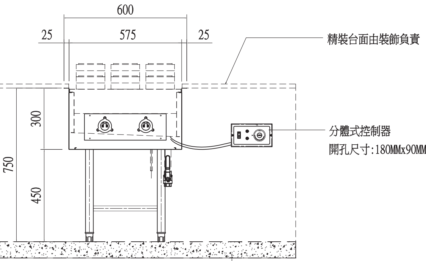
ELEVATION
