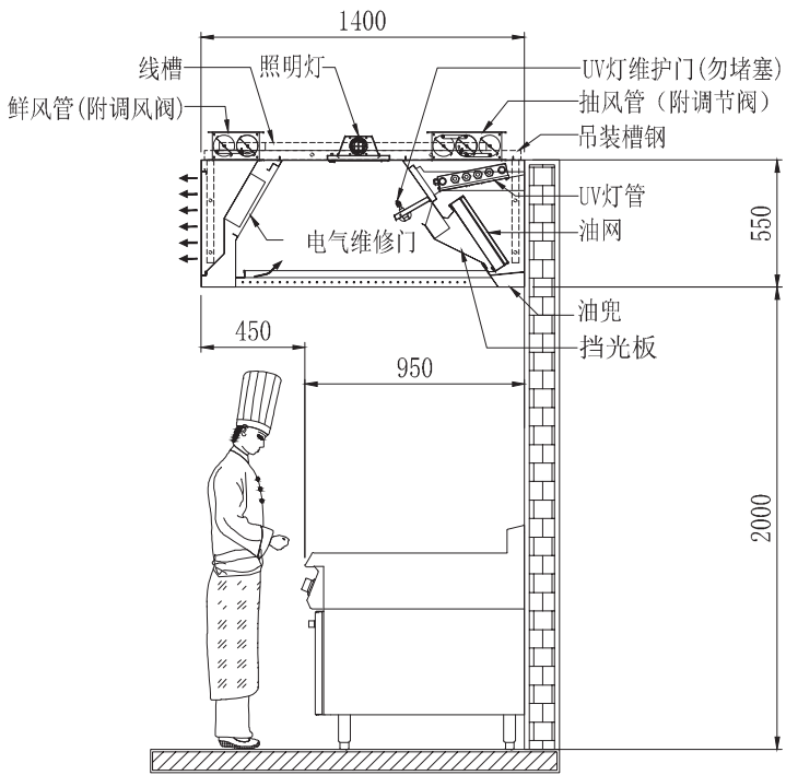
截面示意图
