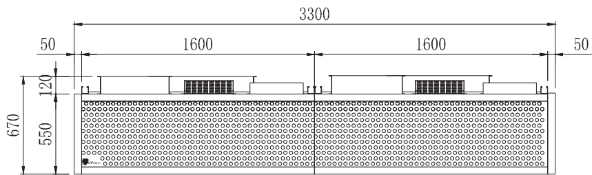
正视图
