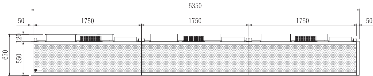
正视图
