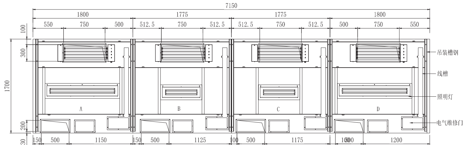
俯视图
