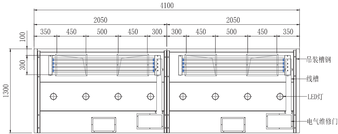
俯视图
