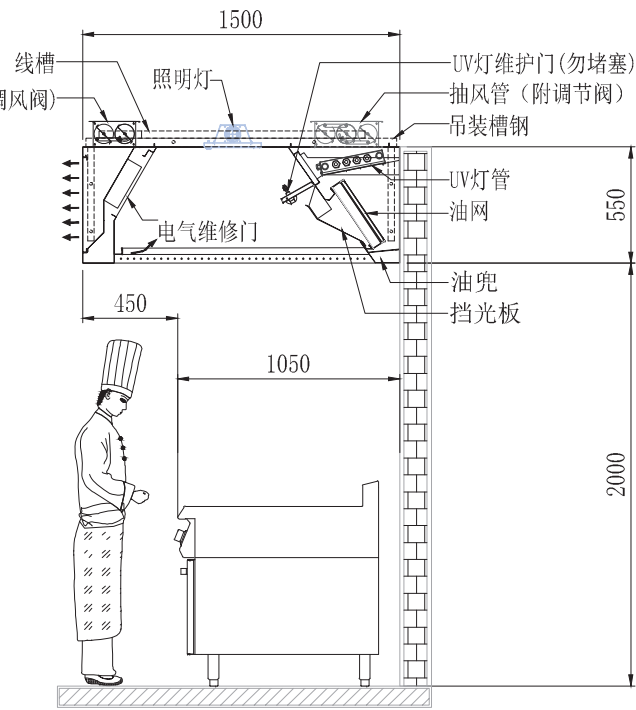
截面示意图
