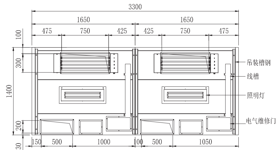
俯视图
