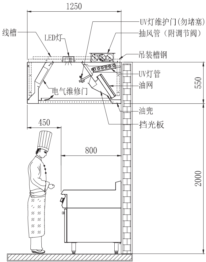
截面示图
