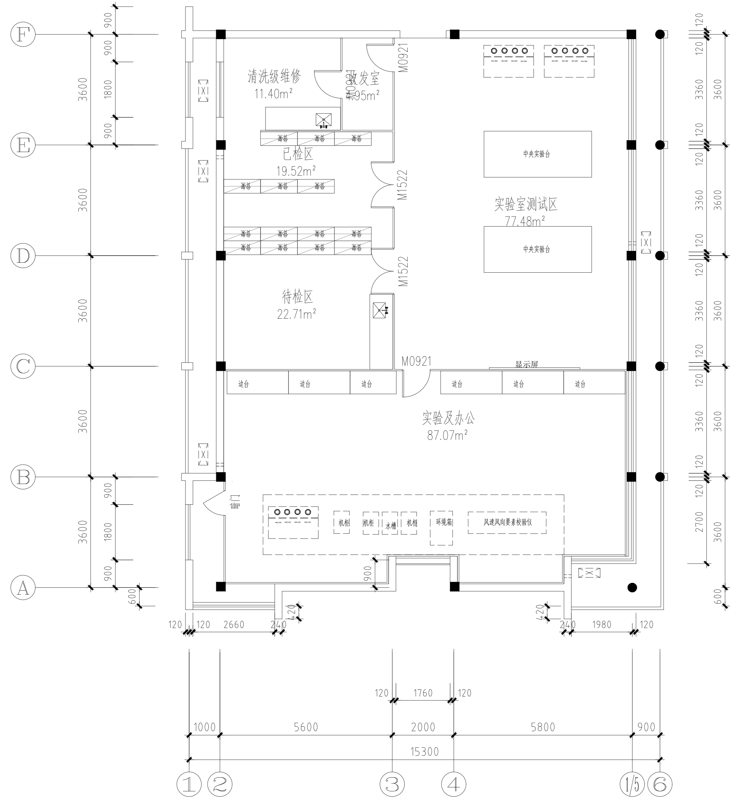
平面图 1:100
