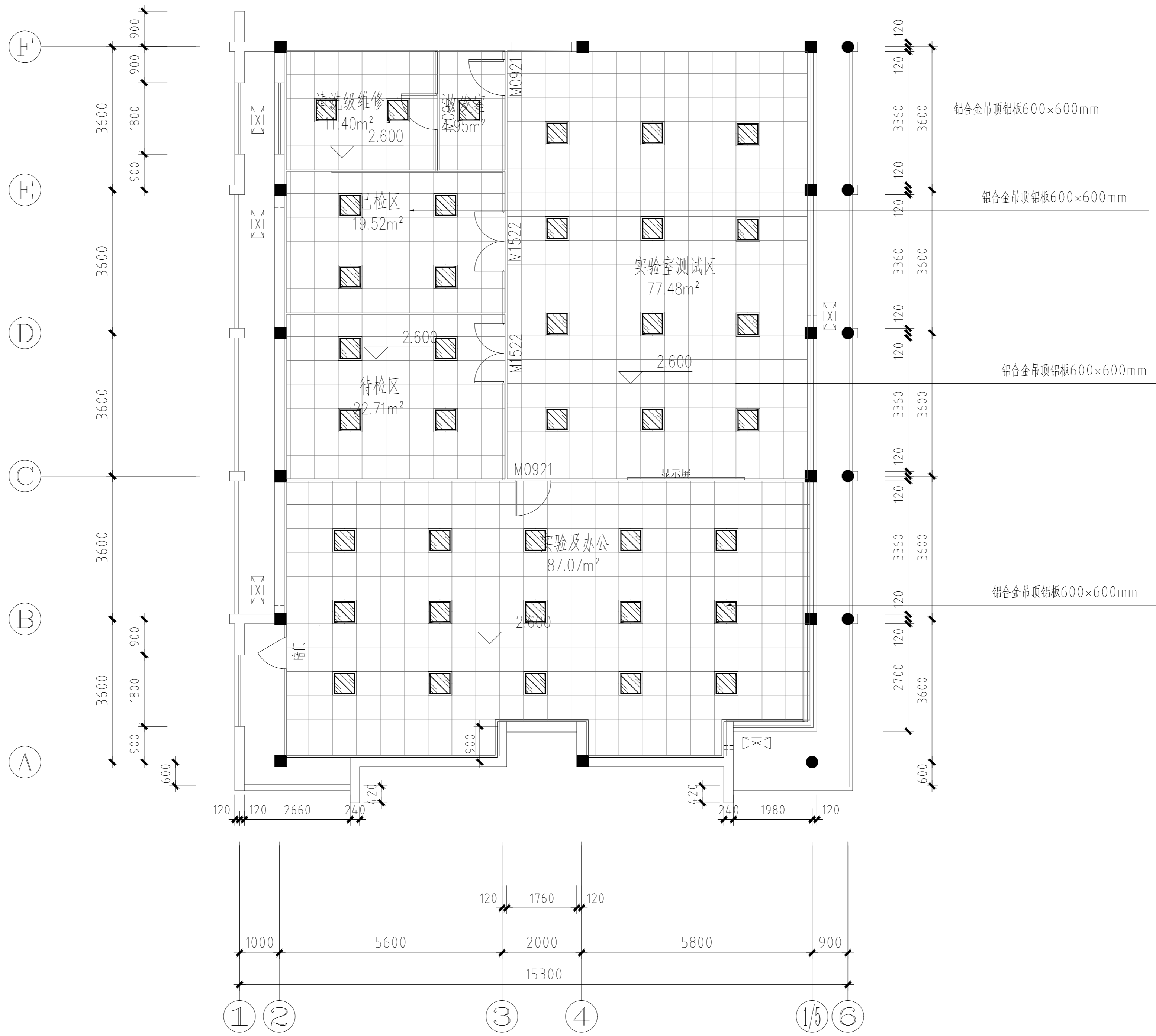
顶面灯具布置图 1:100
