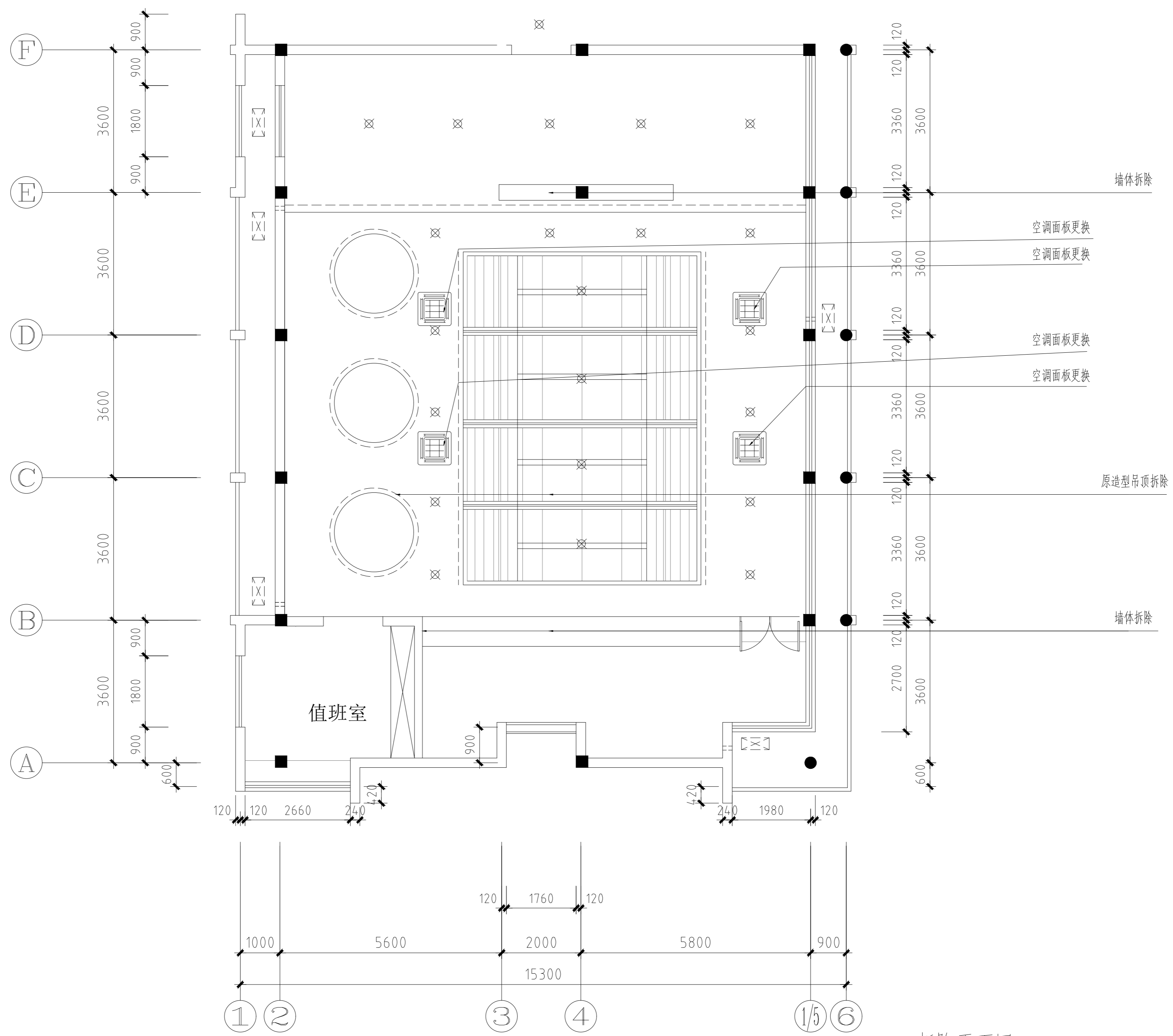
拆除平面图 1:100
