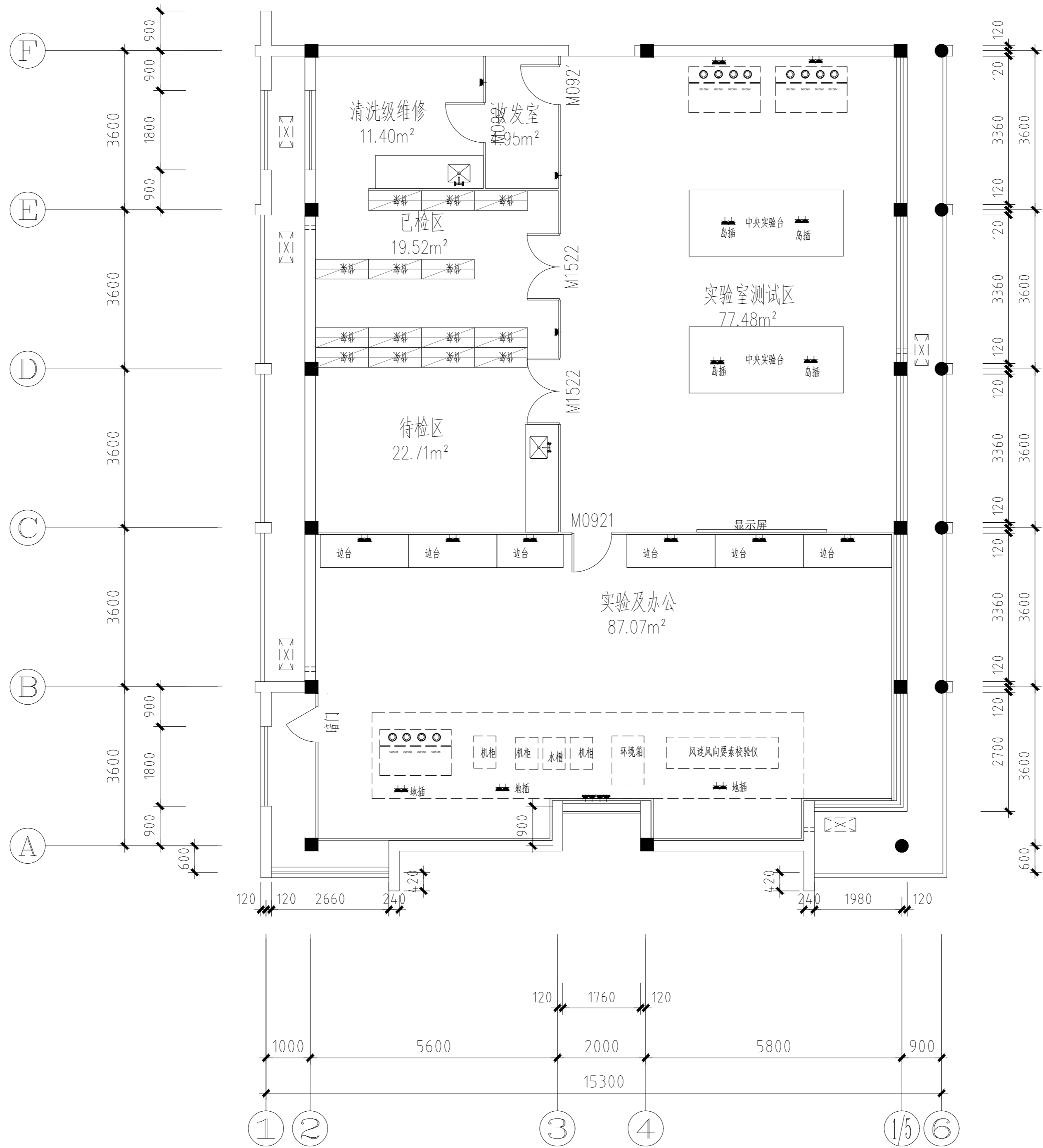
插座点位图 1:100
