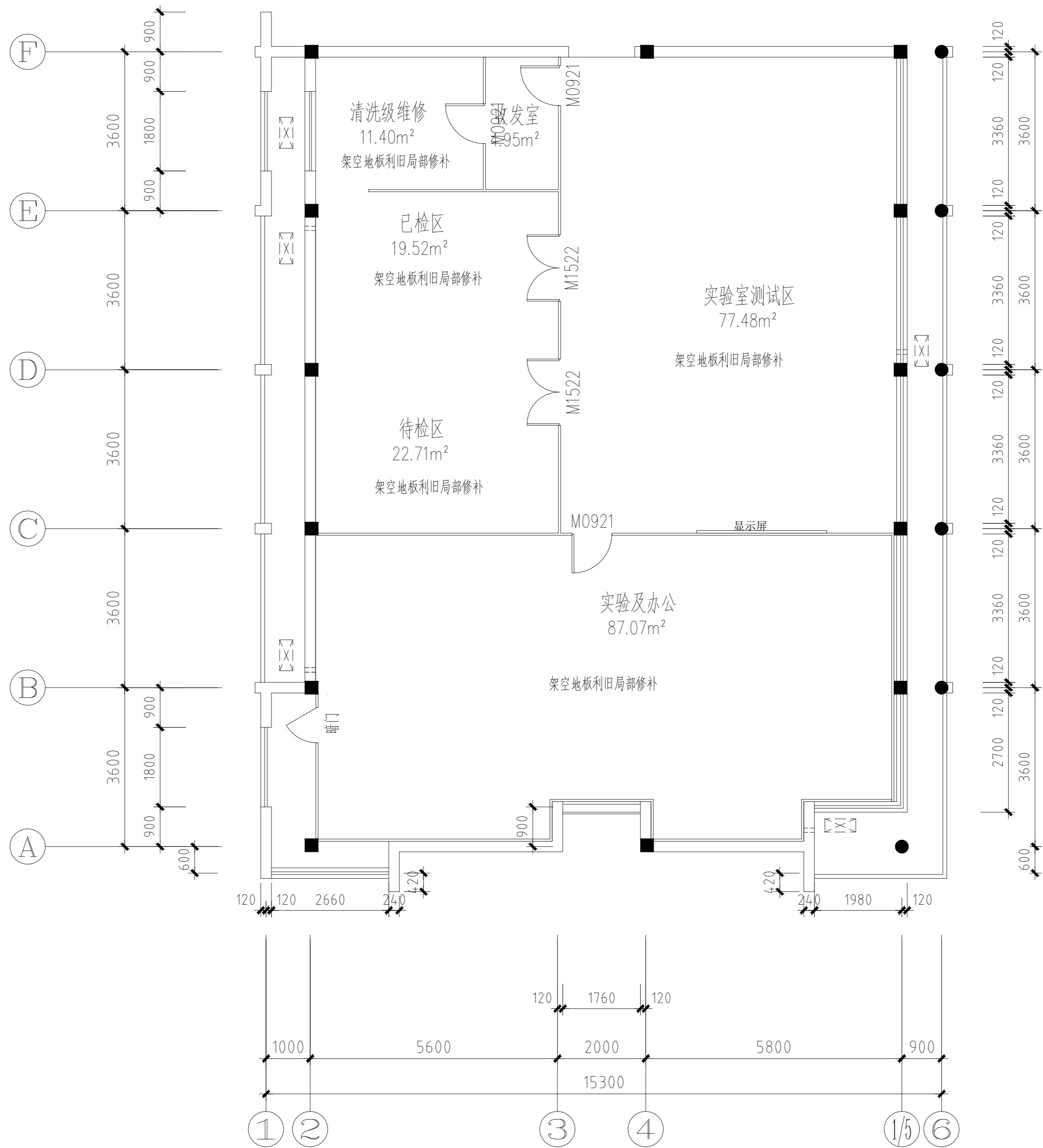
地面布置图 1:100
