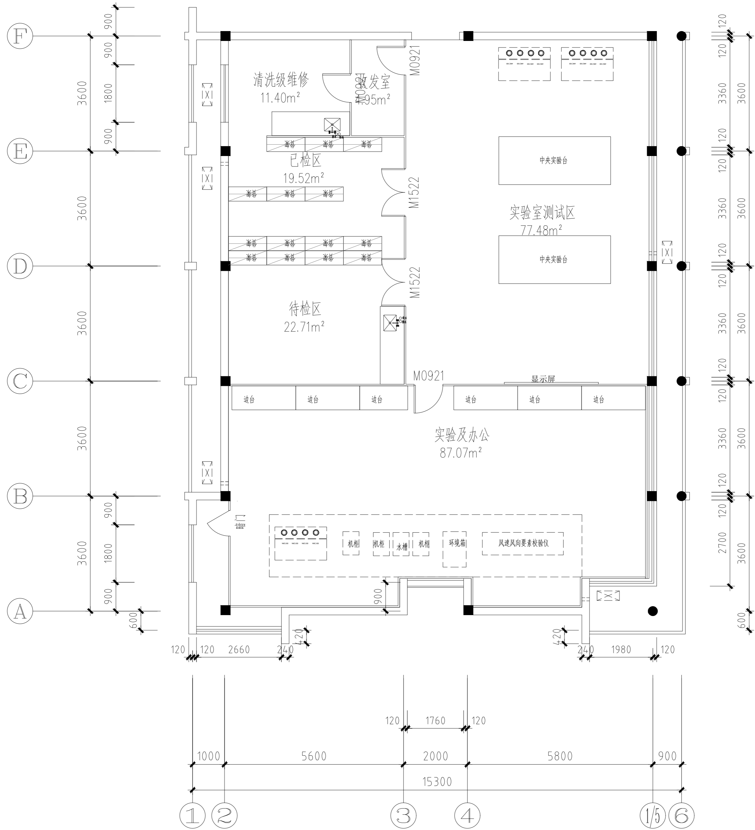
给排水点位图 1:100
