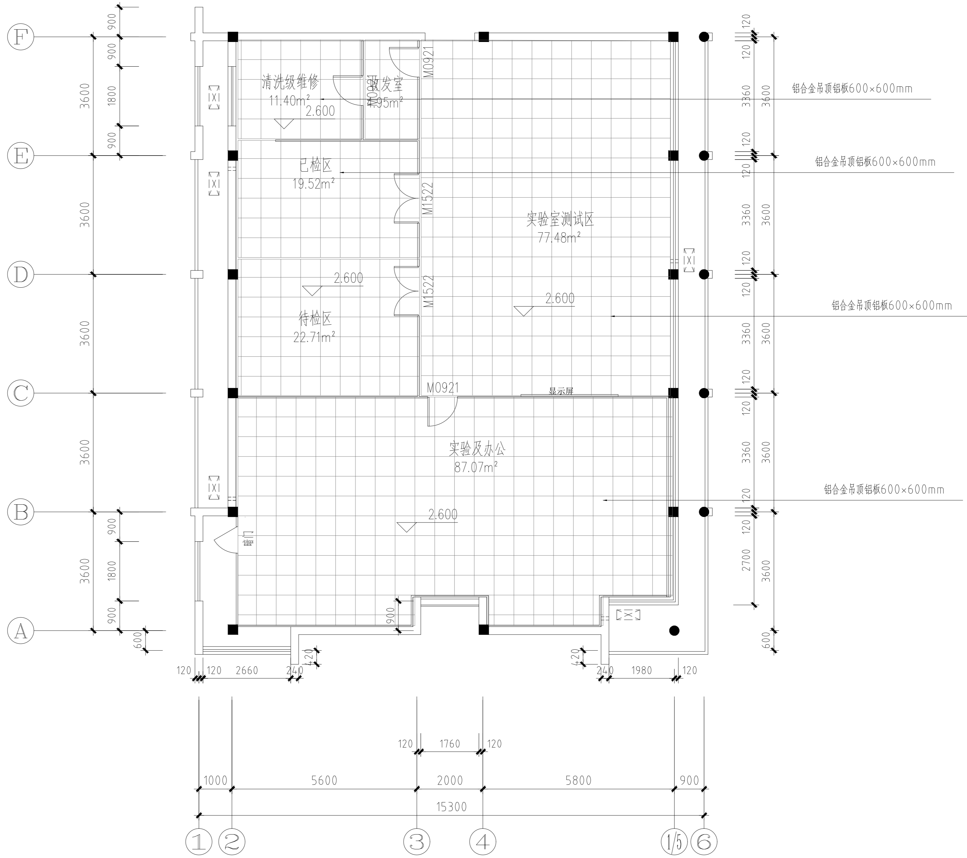
顶面布置图 1:100
