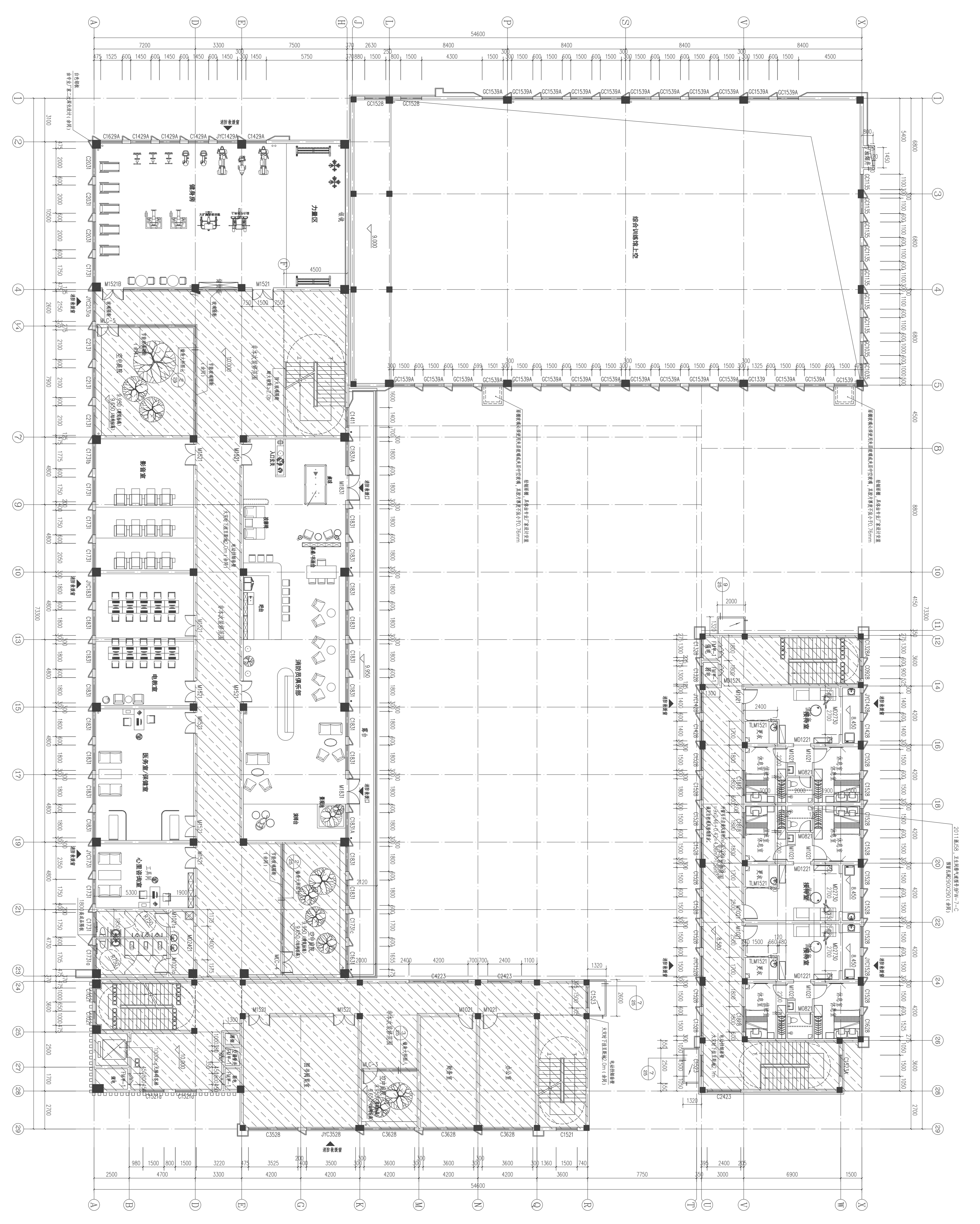
三层平面图 1:100
