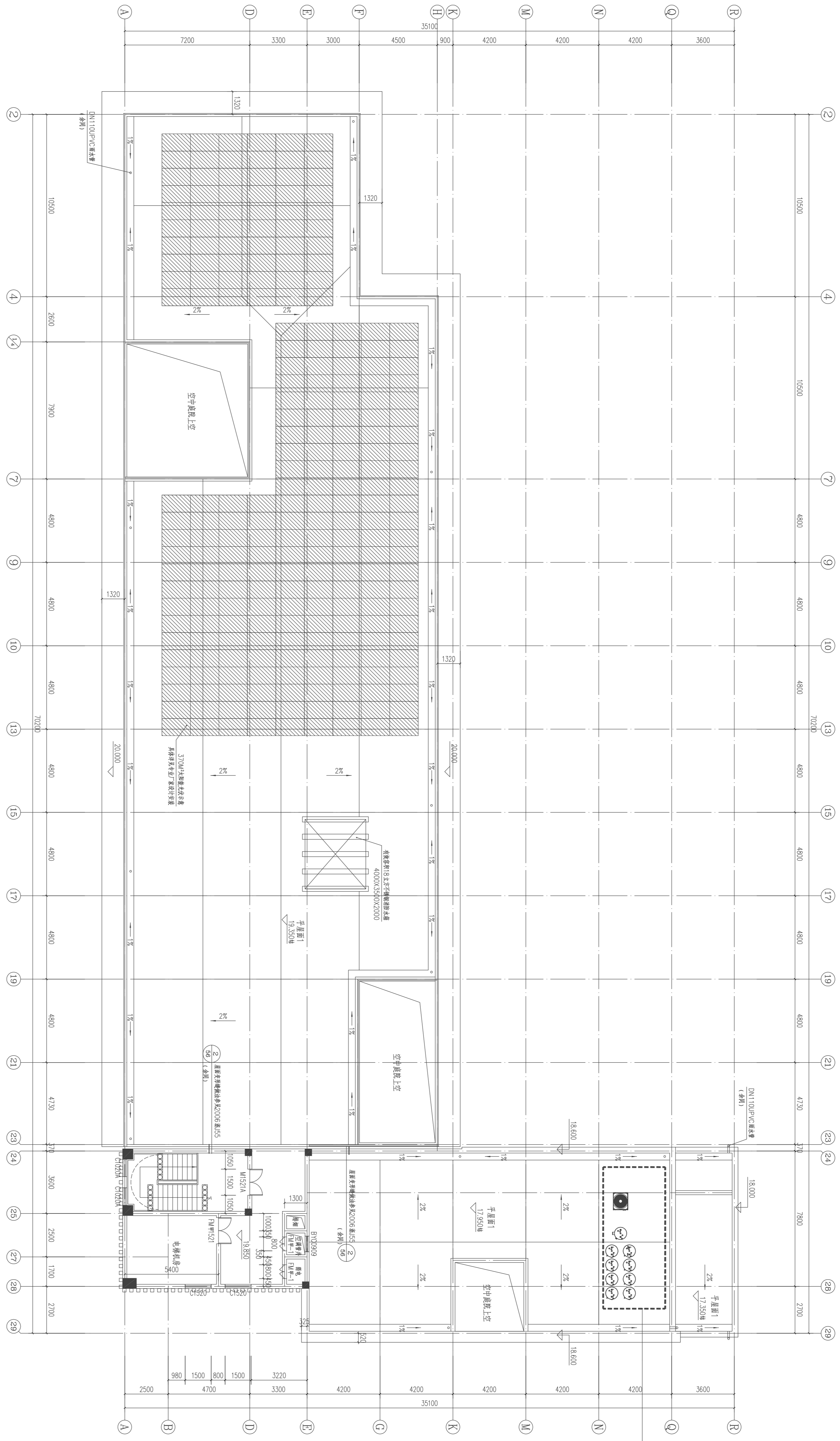
屋顶层平面图 1:100
