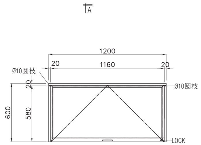
ELEVATION 01
