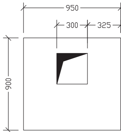
PLAN (俯视图)
