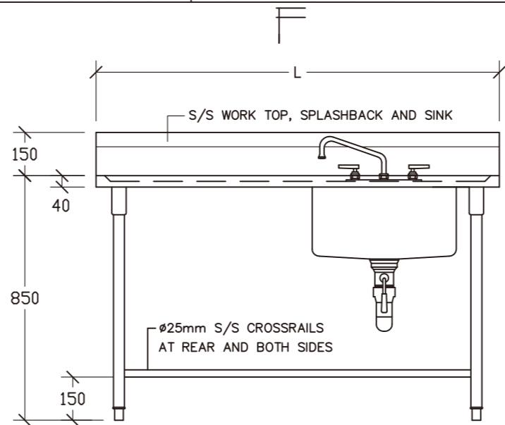
ELEVATION
