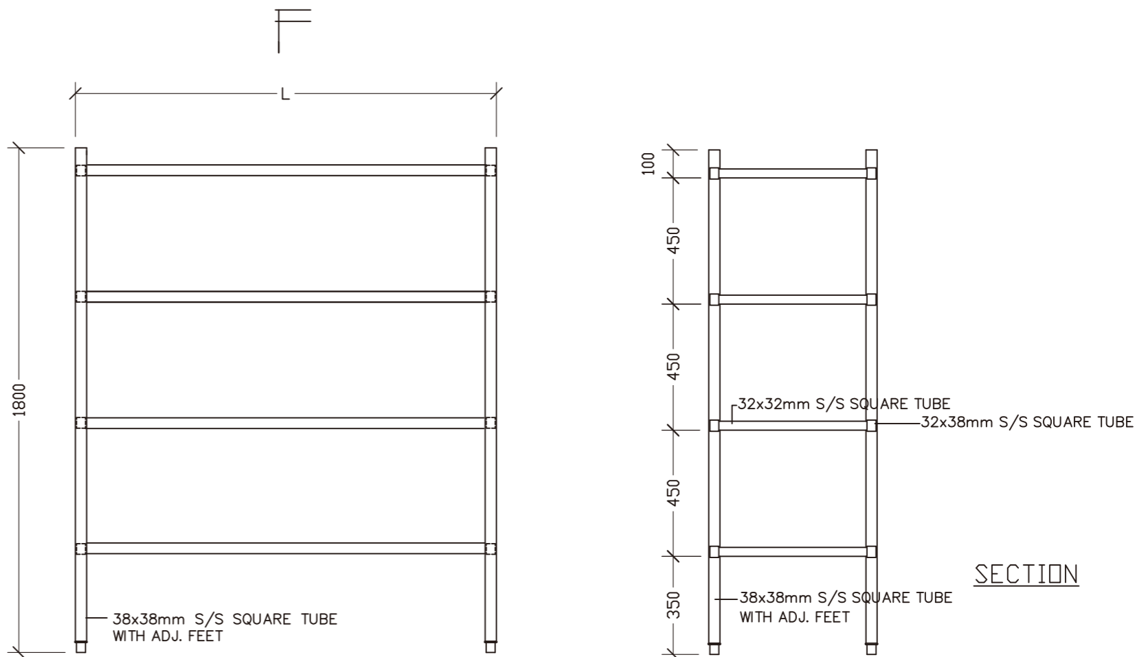
ELEVATION
