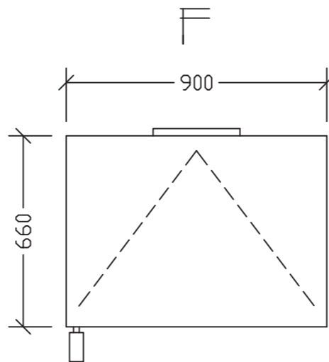
ELEVATION (主视图)
