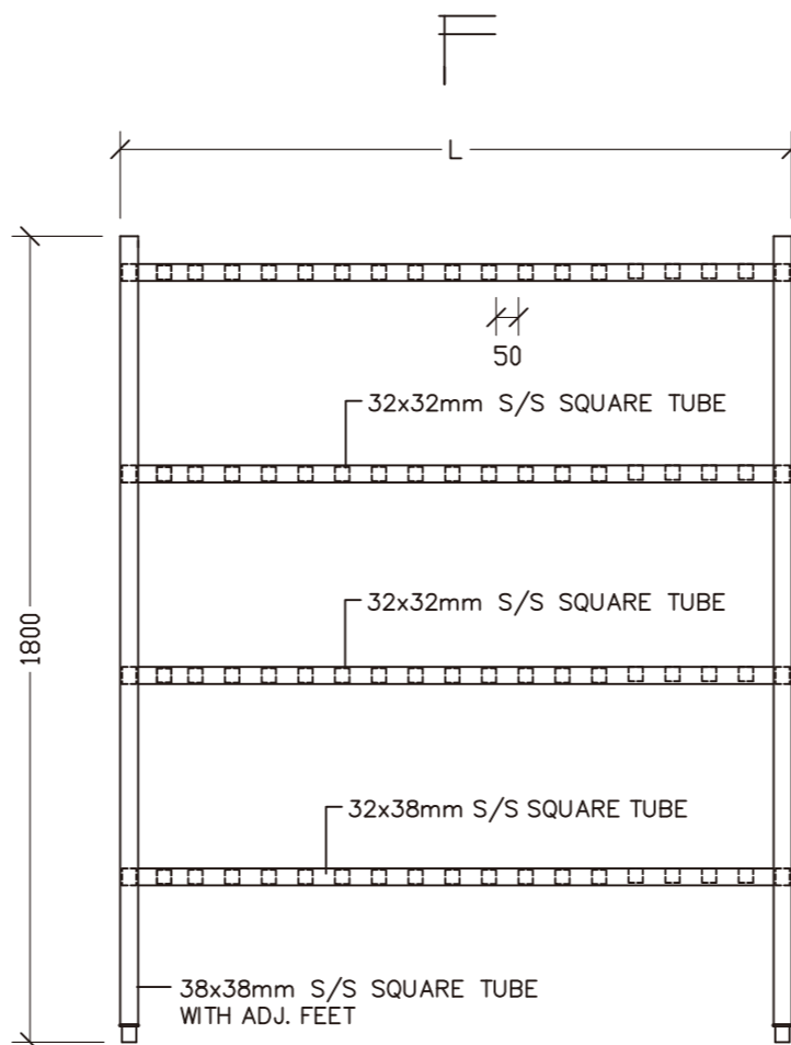
ELEVATION
