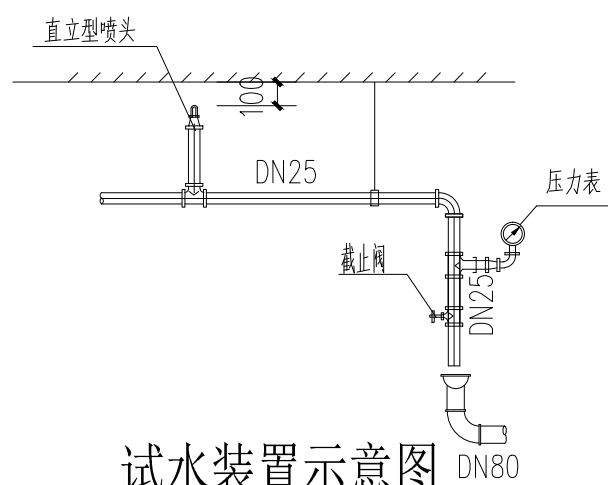
试水装置示意图
