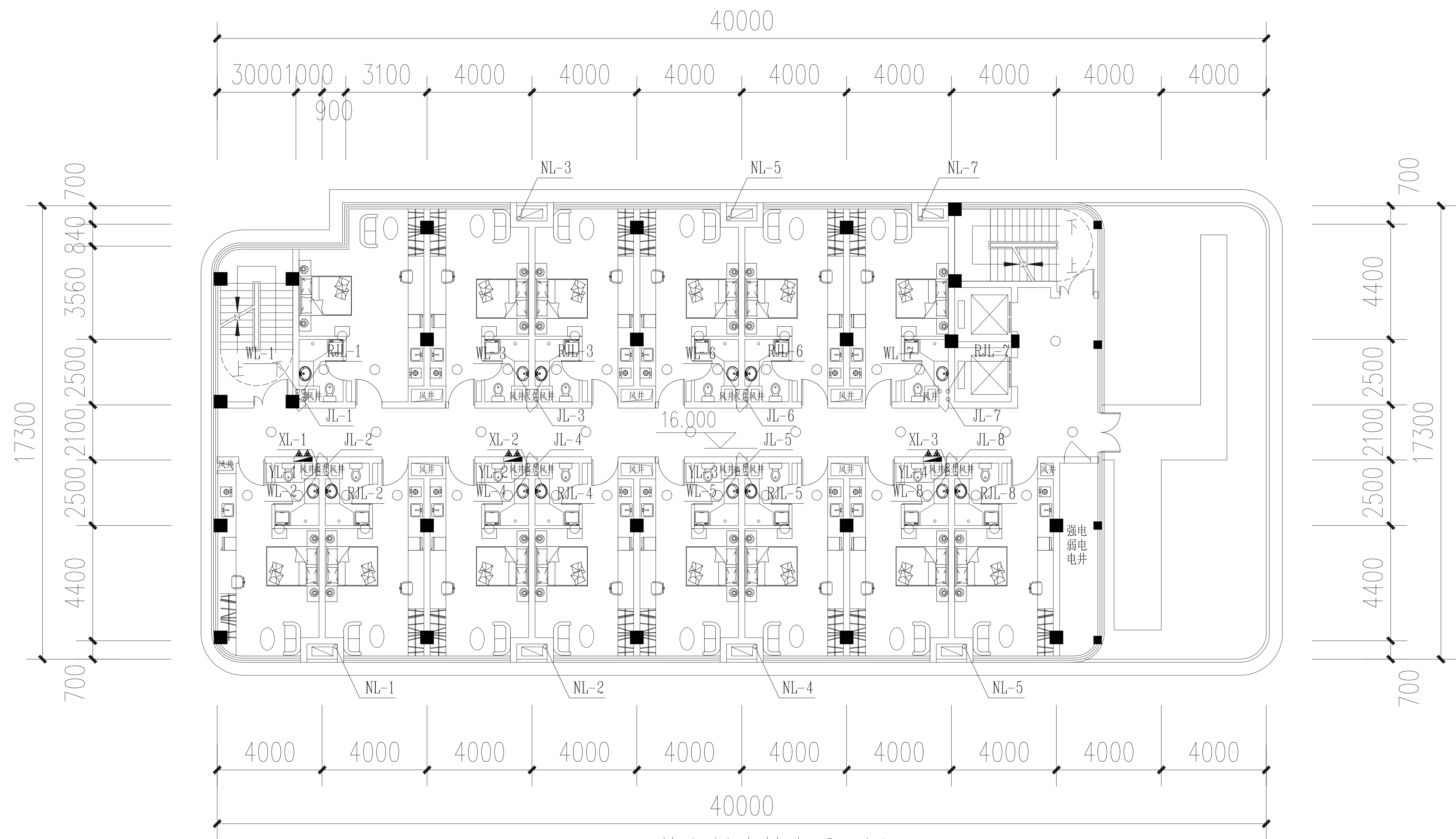
6#楼六层给排水平面图 1:200
