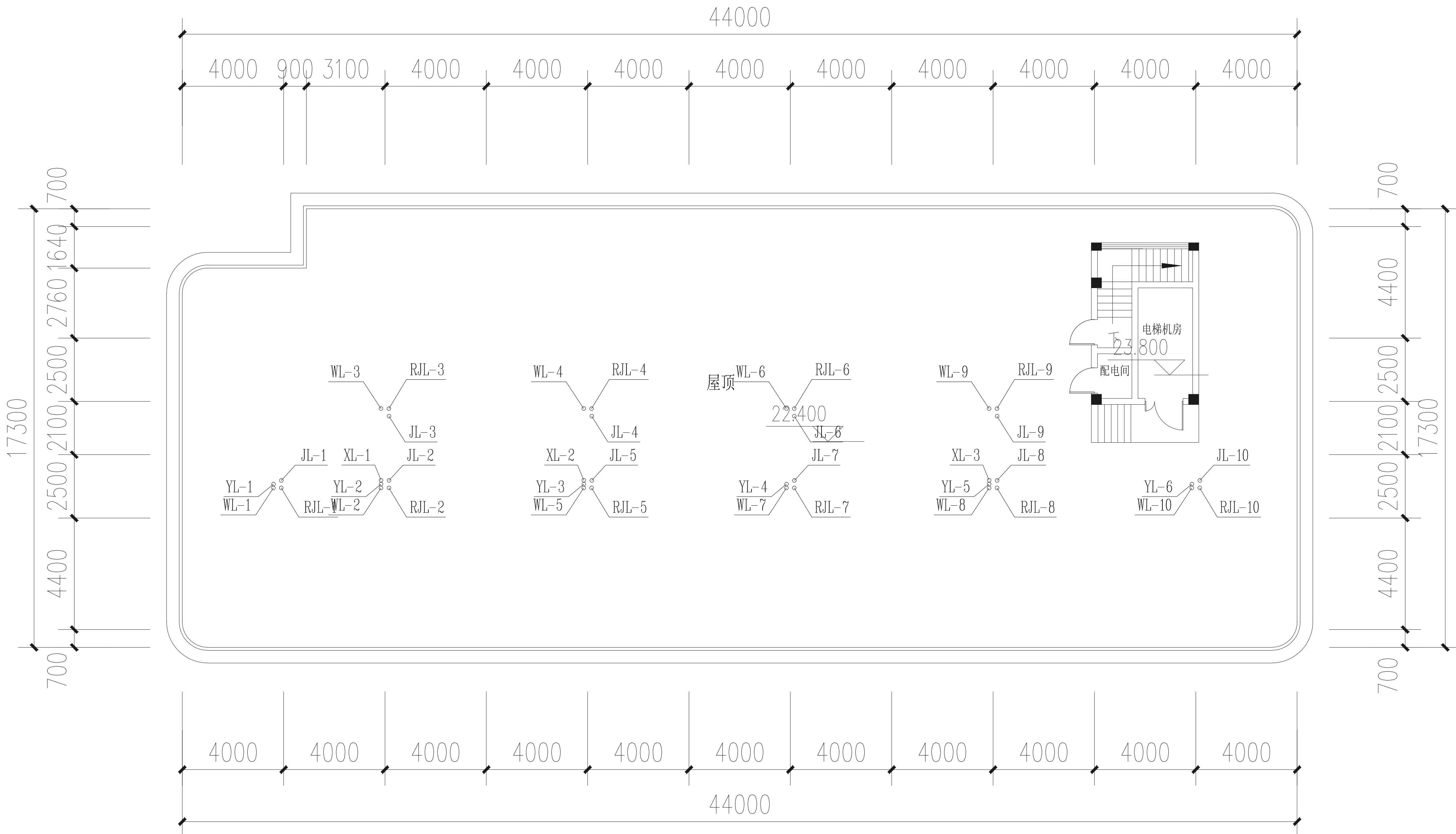
7#楼机房层给排水平面图 1:200
