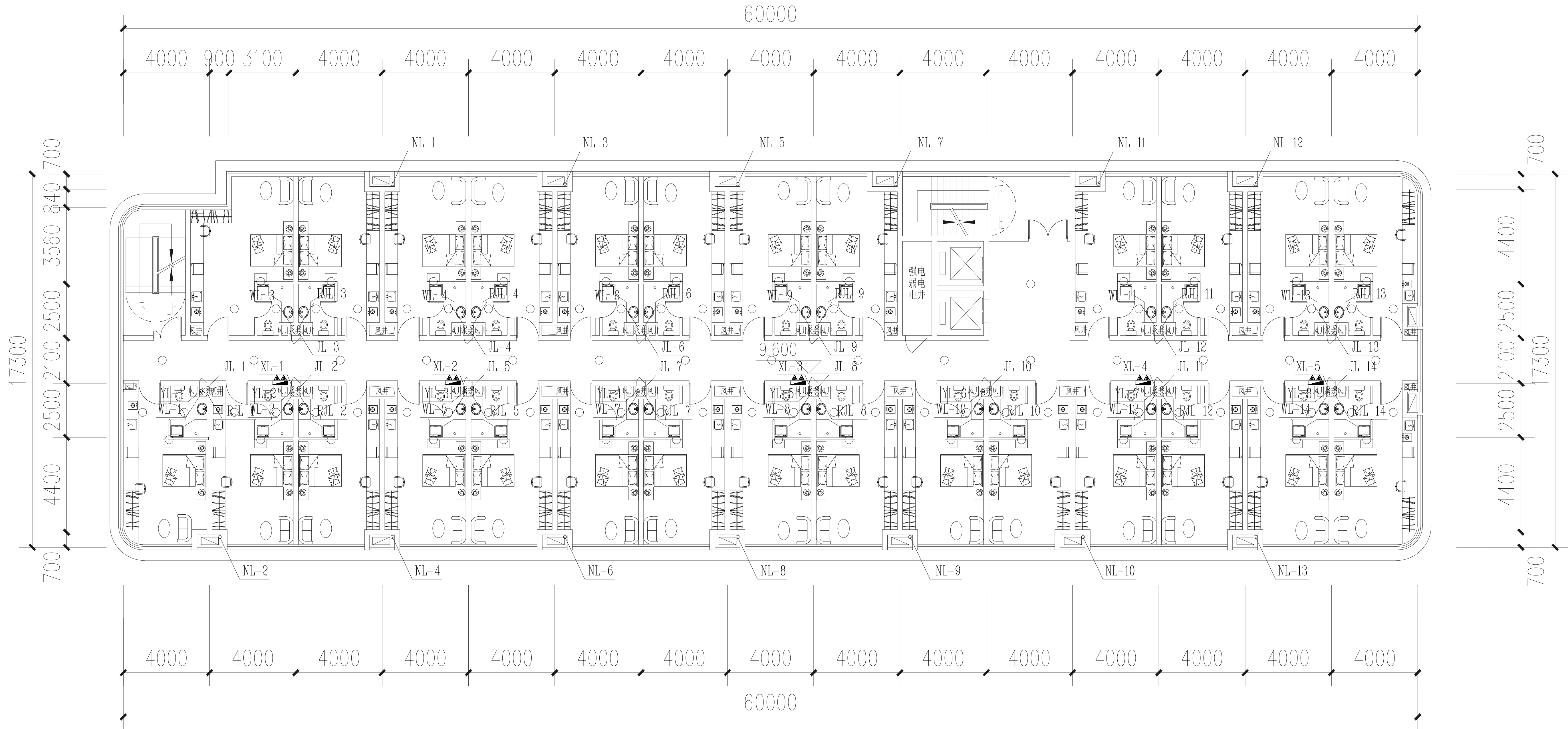
7#楼四层给排水平面图 1:200
