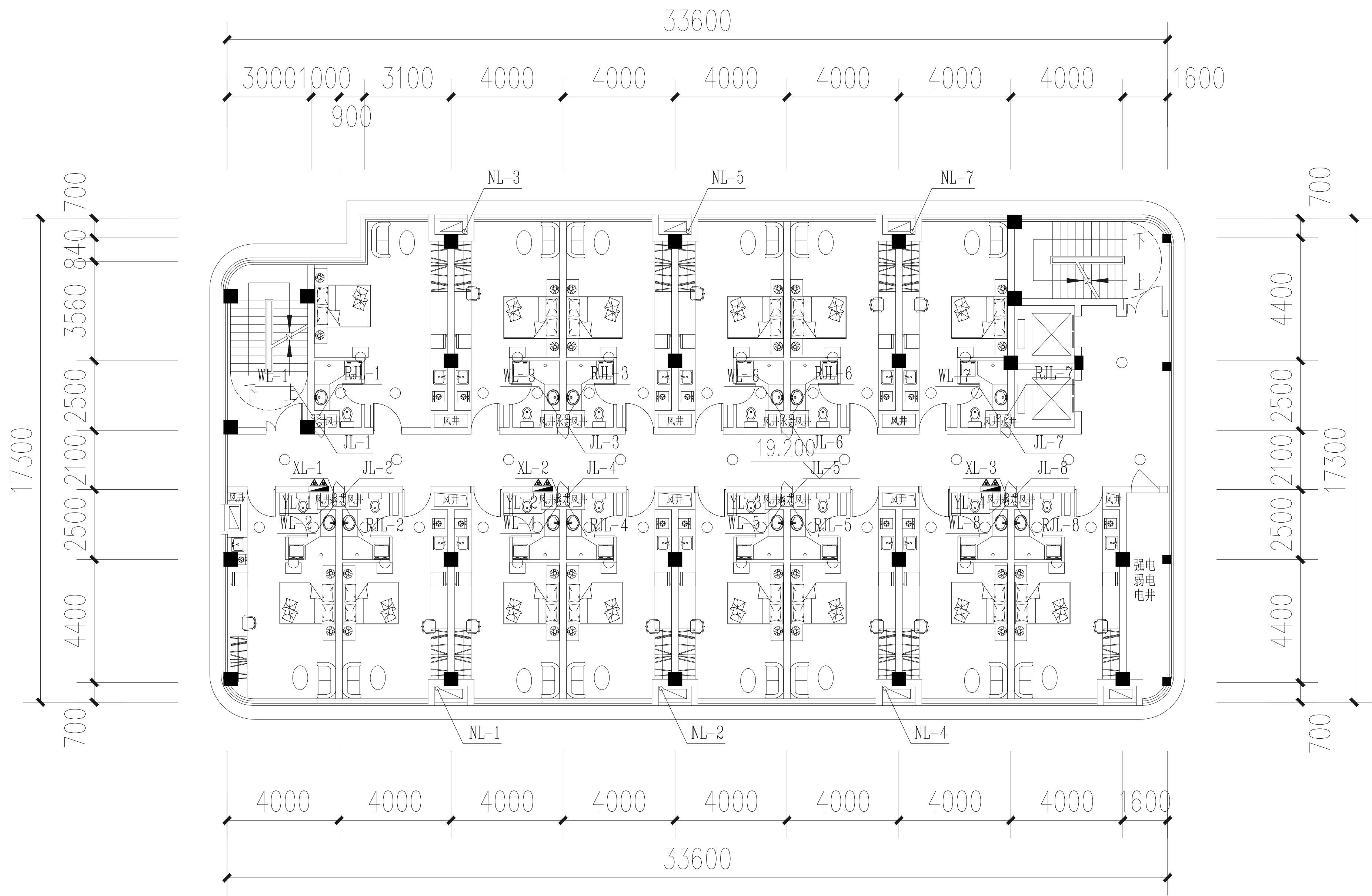
6#楼七层给排水平面图 1:200
