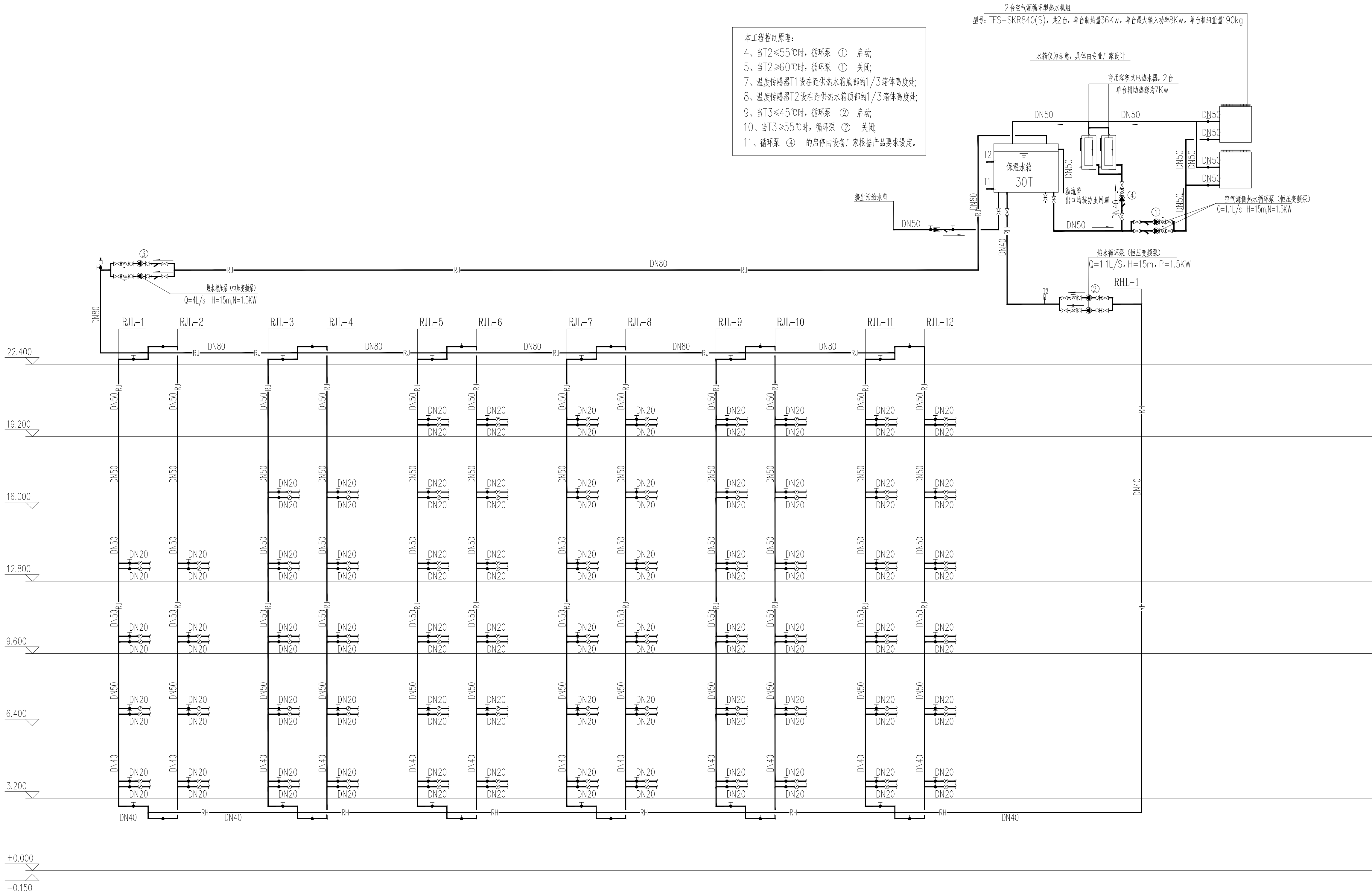
热水系统原理图
