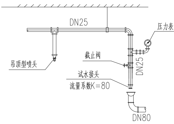
末端试水装置示意图
