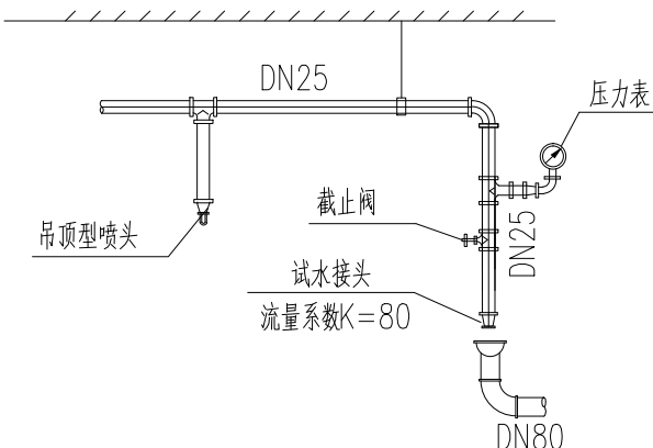
末端试水装置示意图
