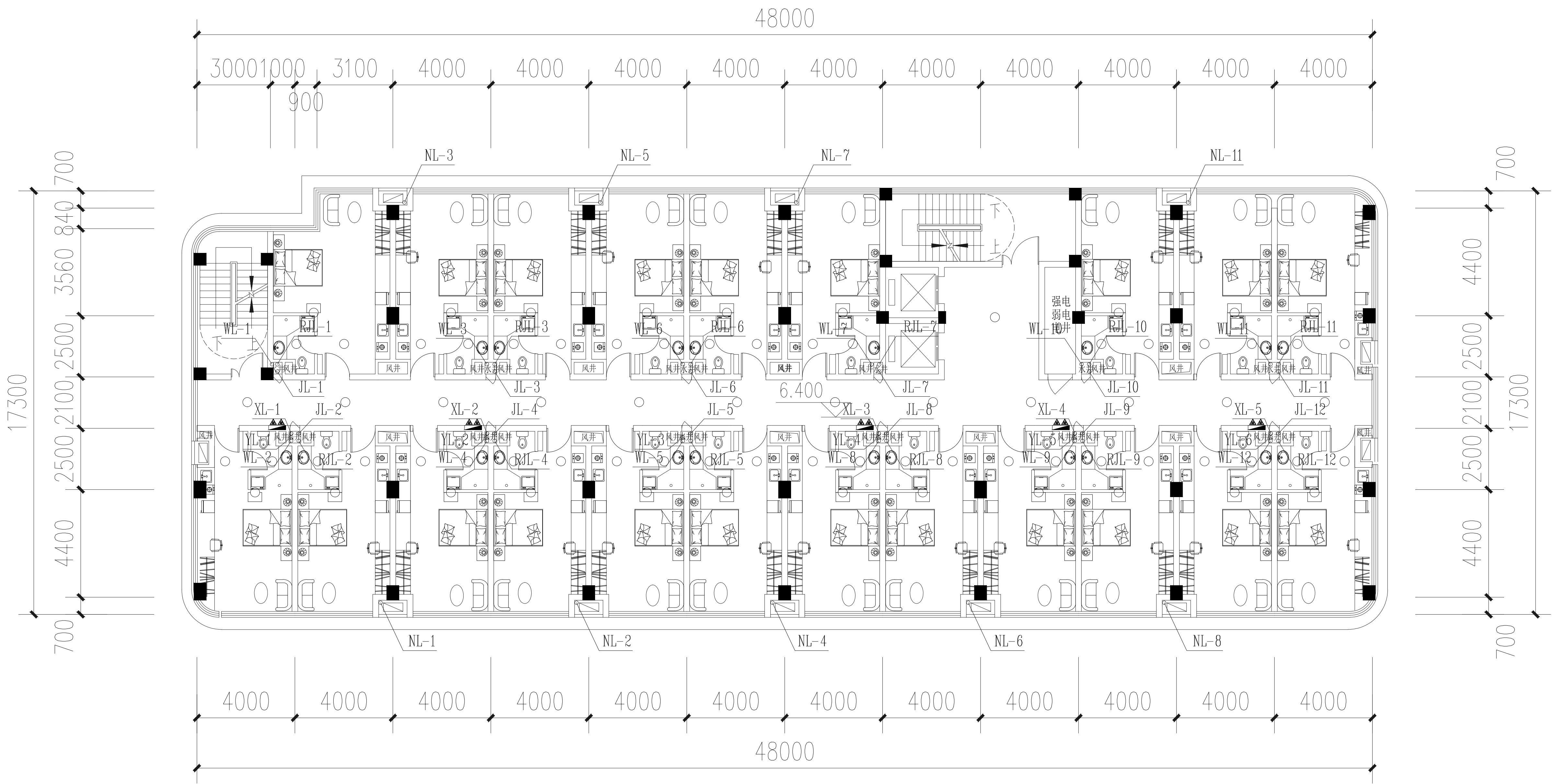
6#楼三层给排水平面图 1:200
