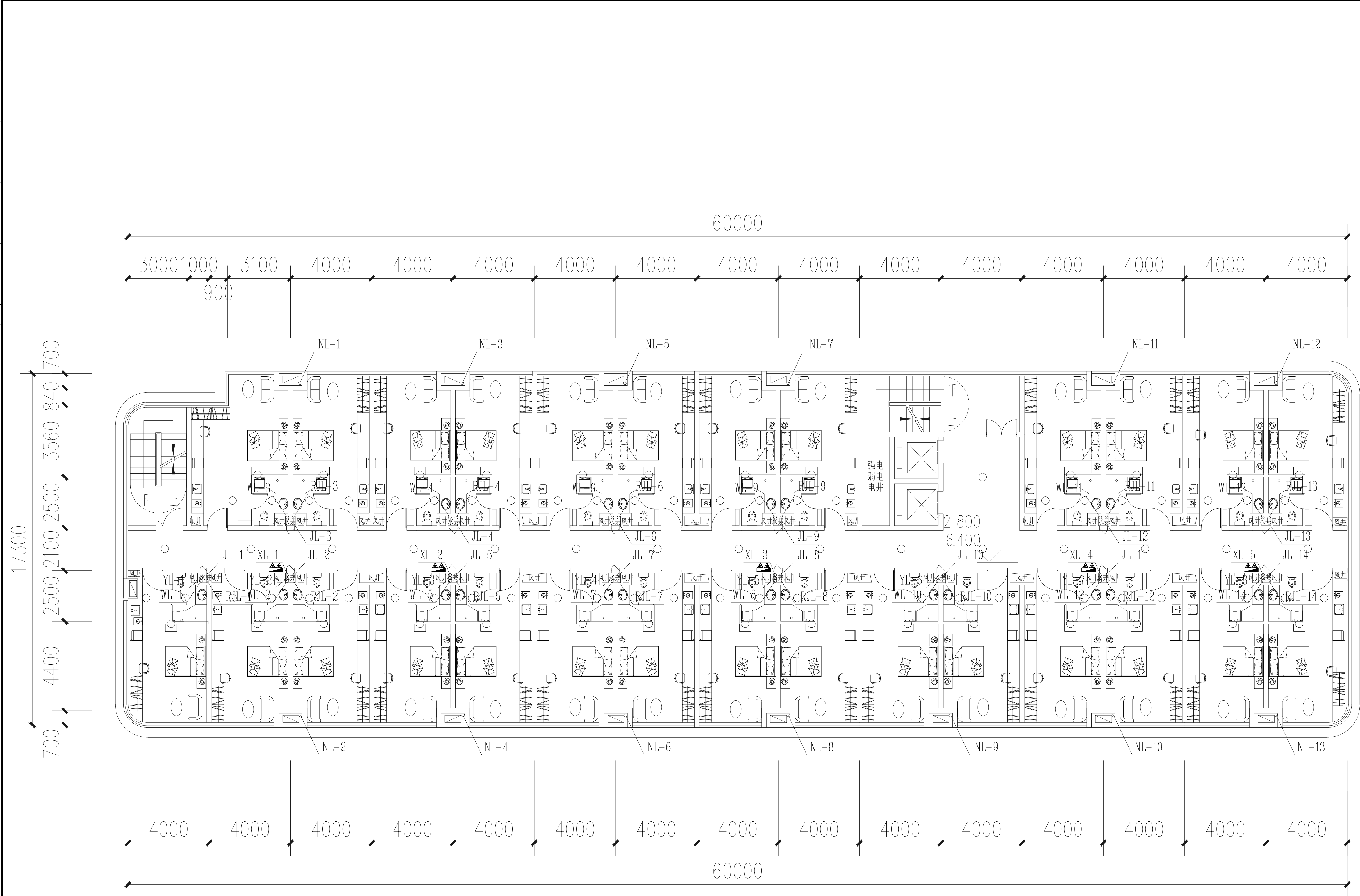
7#楼三、五层给排水平面图 1:200
