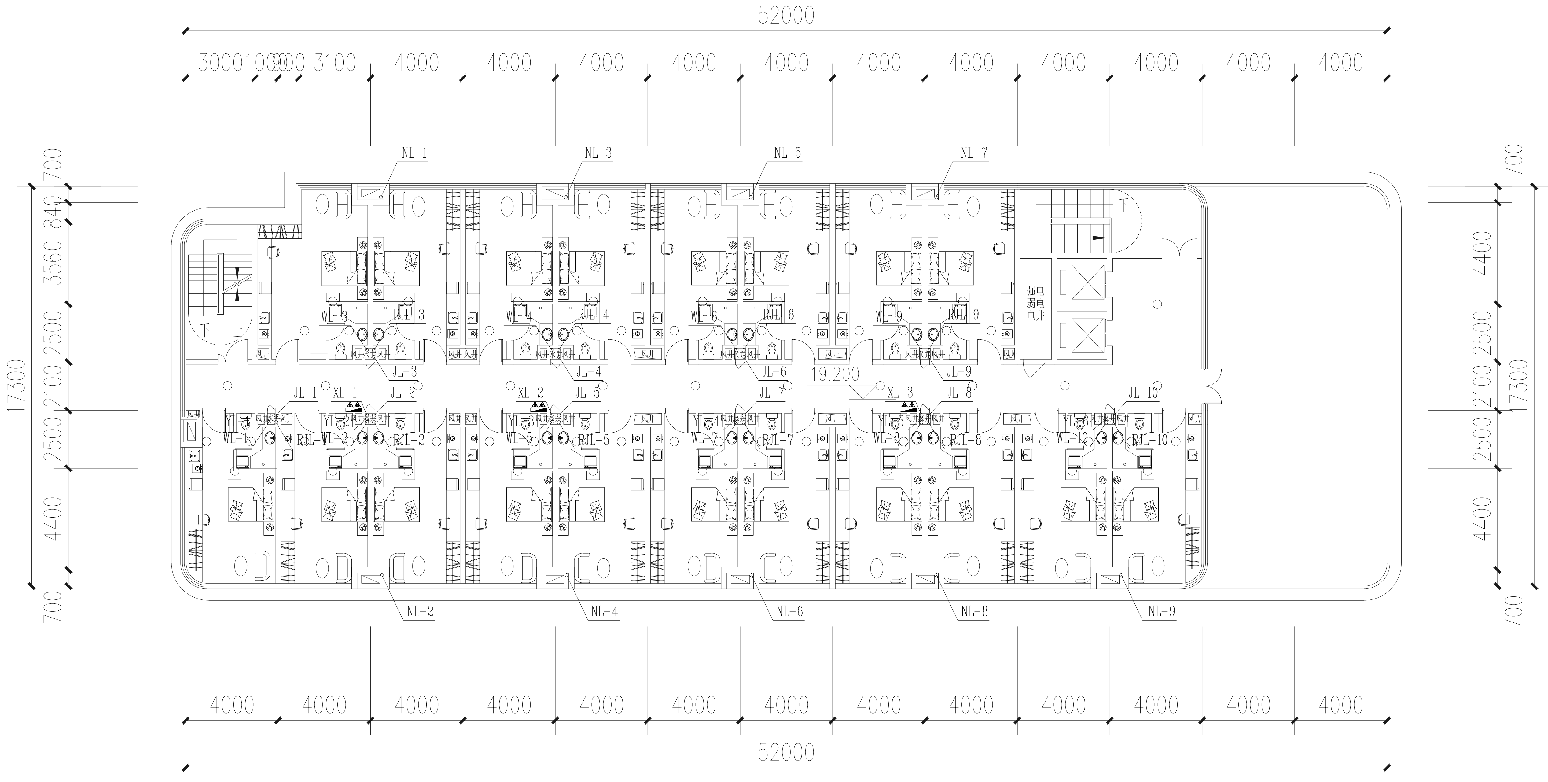
7#楼七层给排水平面图 1:200
