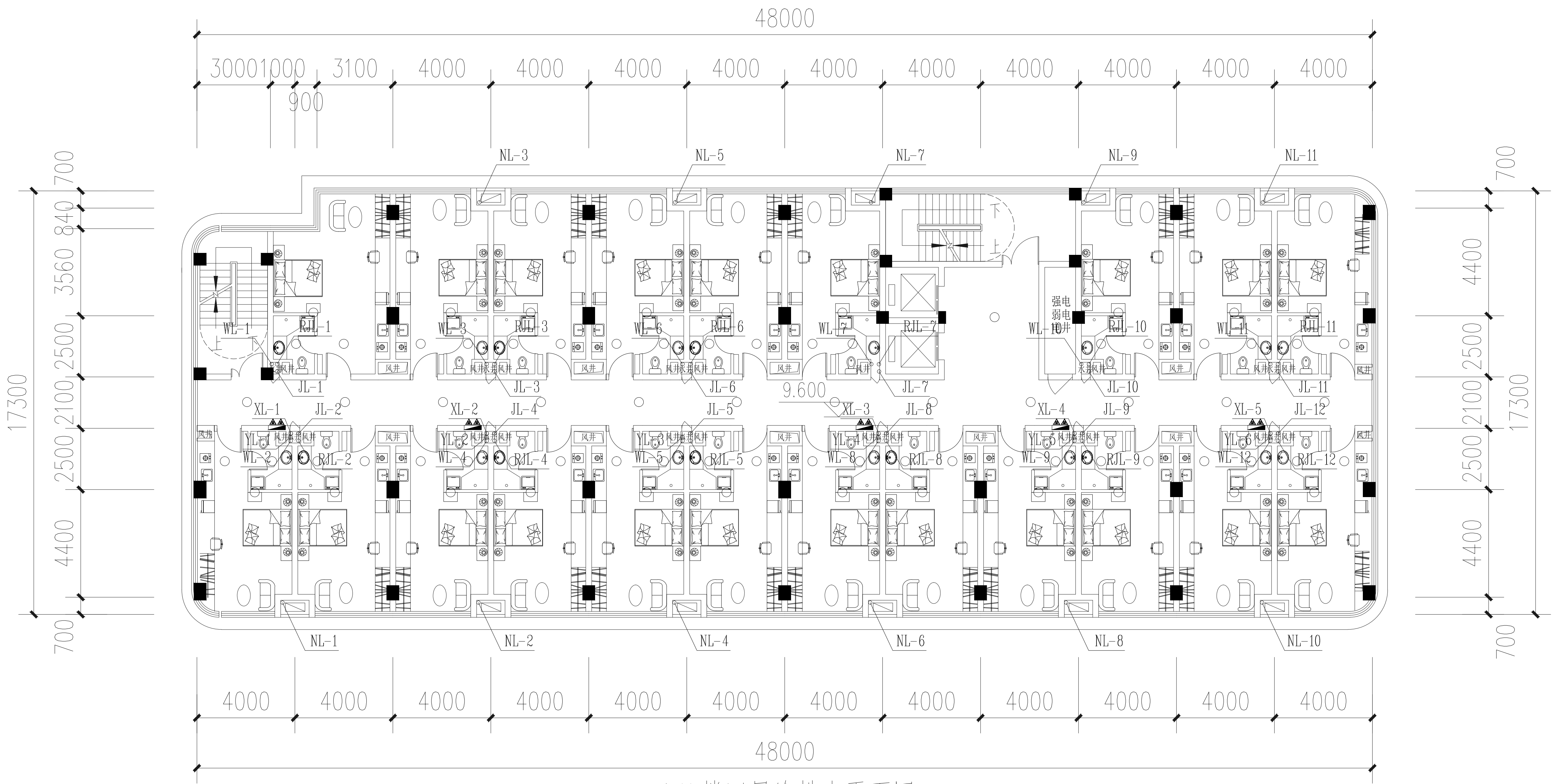
6#楼四层给排水平面图 1:200
