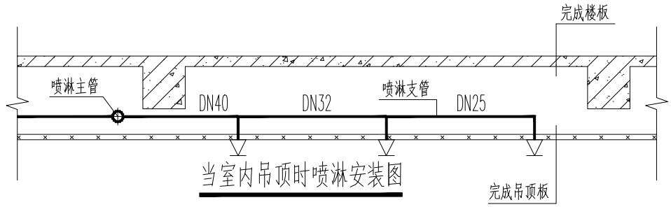
当室内吊顶时喷淋安装图
