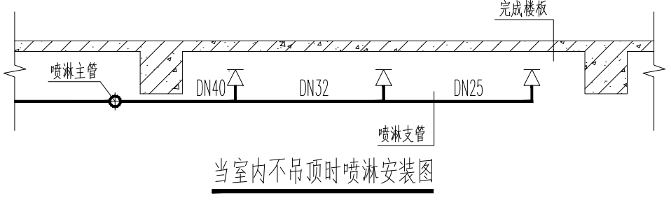
当室内不吊顶时喷淋安装图
