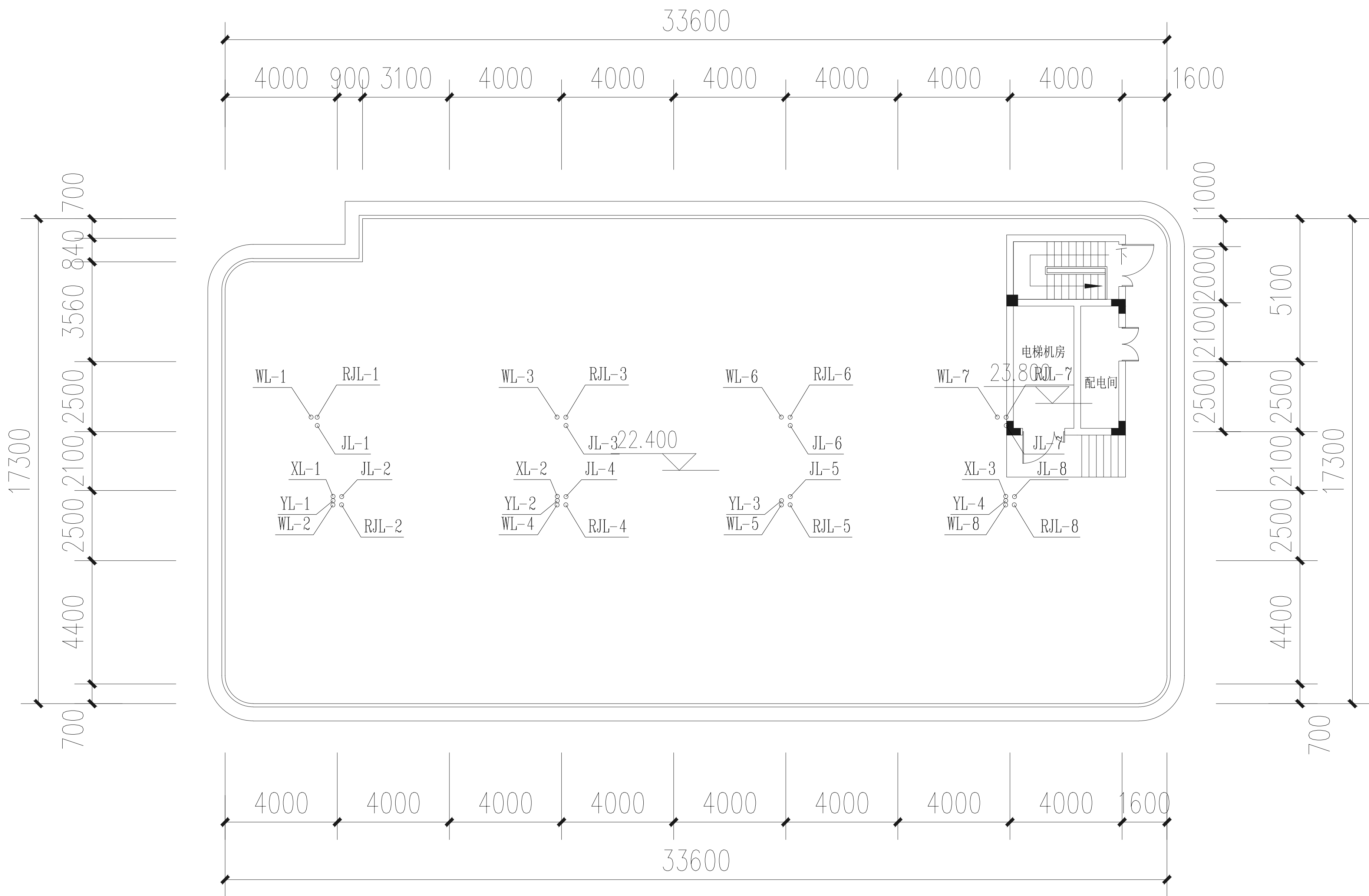
6#楼机房层给排水水平面图 1:200
