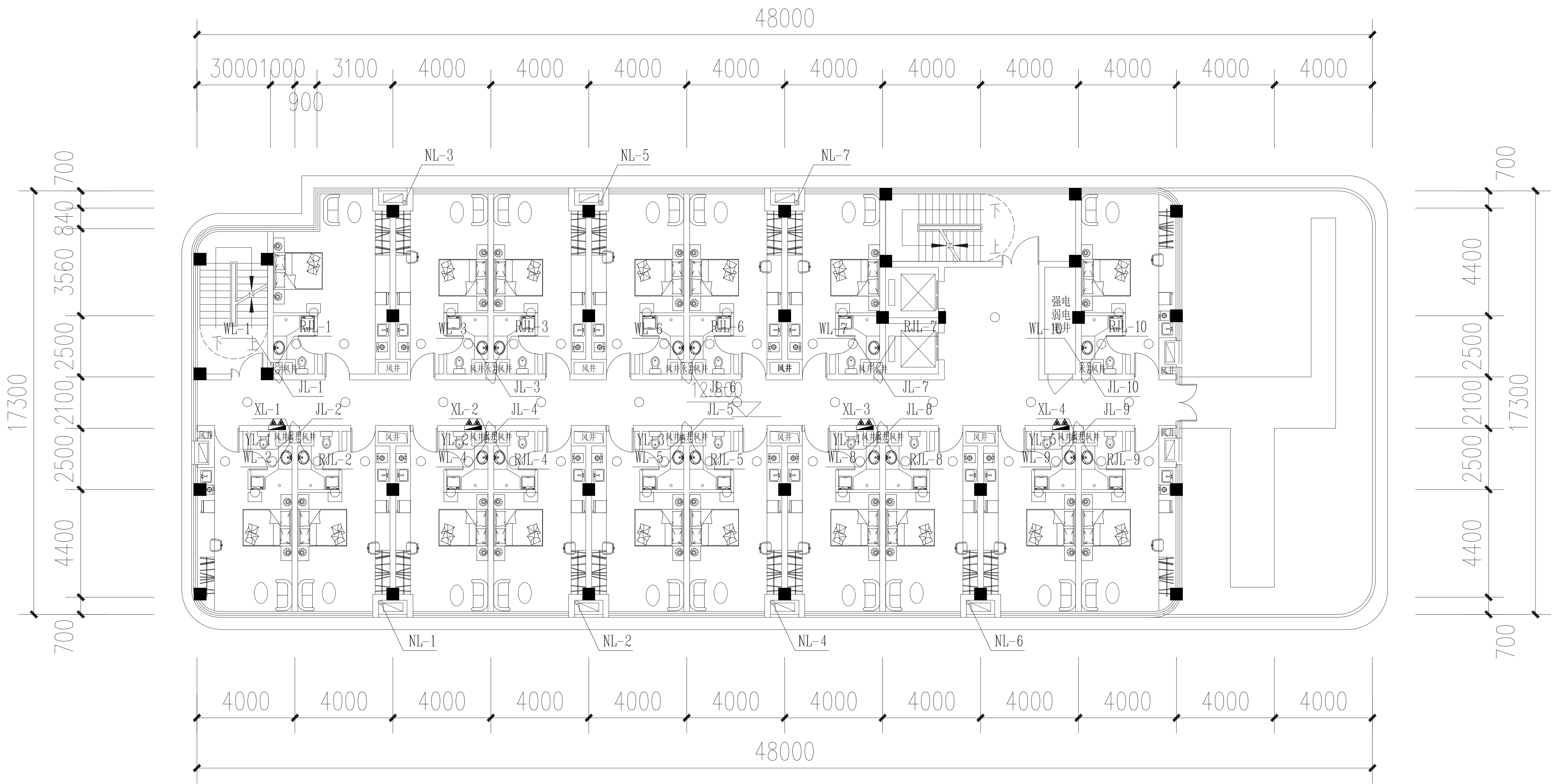
6#楼五层给排水平面图 1:200
