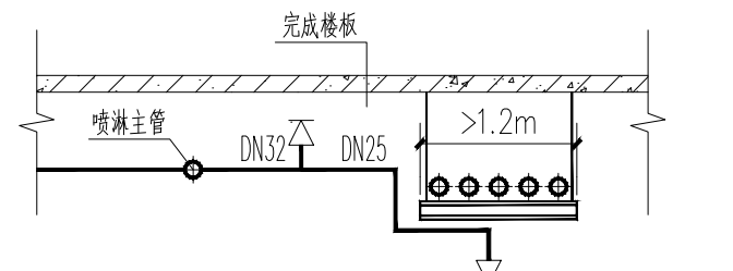
当梁、风管、成排布置的管道、桥架等障碍物大于1.2米时
