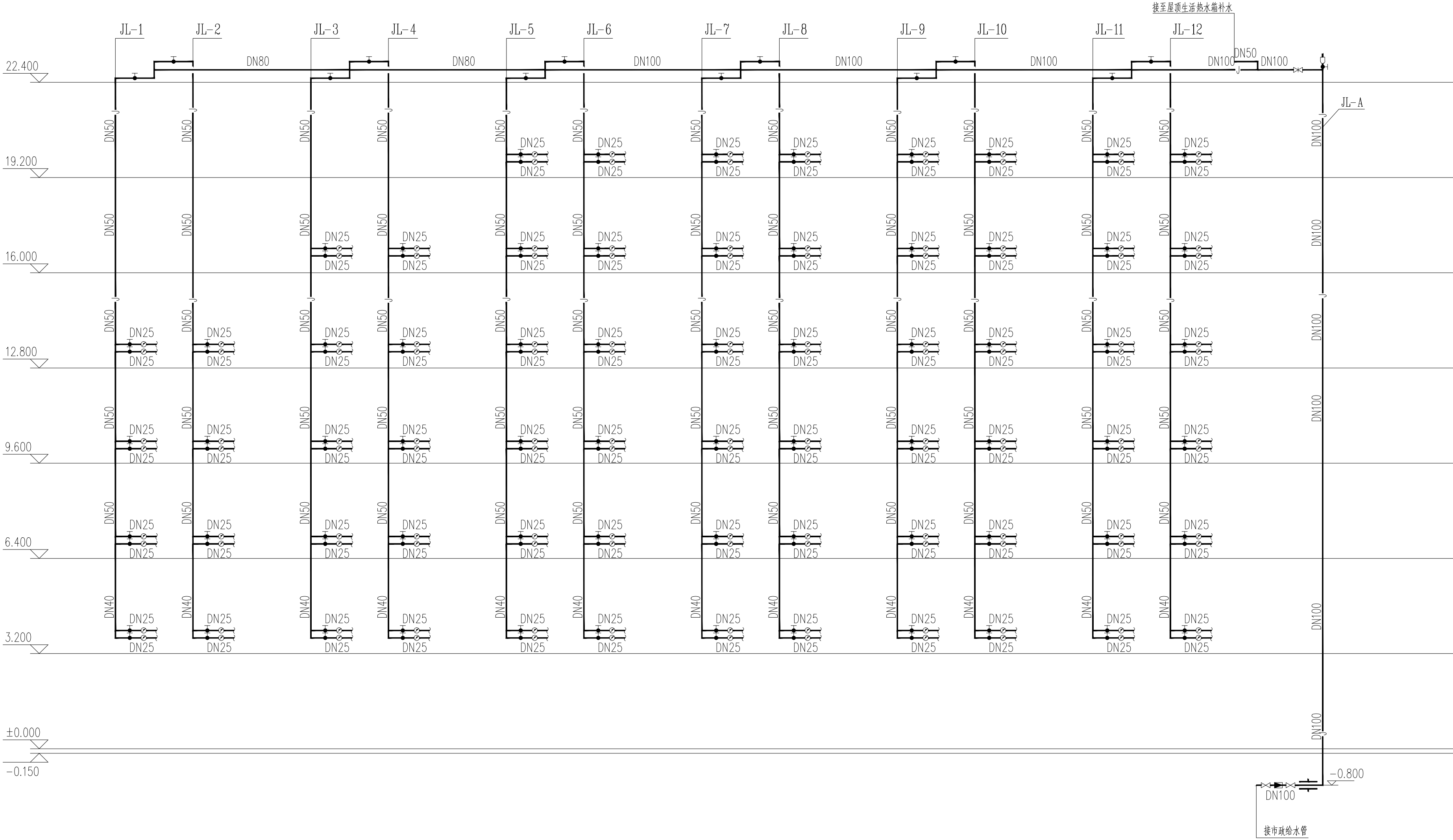
冷水系统原理图
