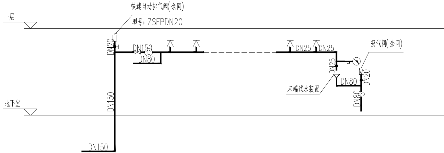
地下车库喷淋系统原理图
