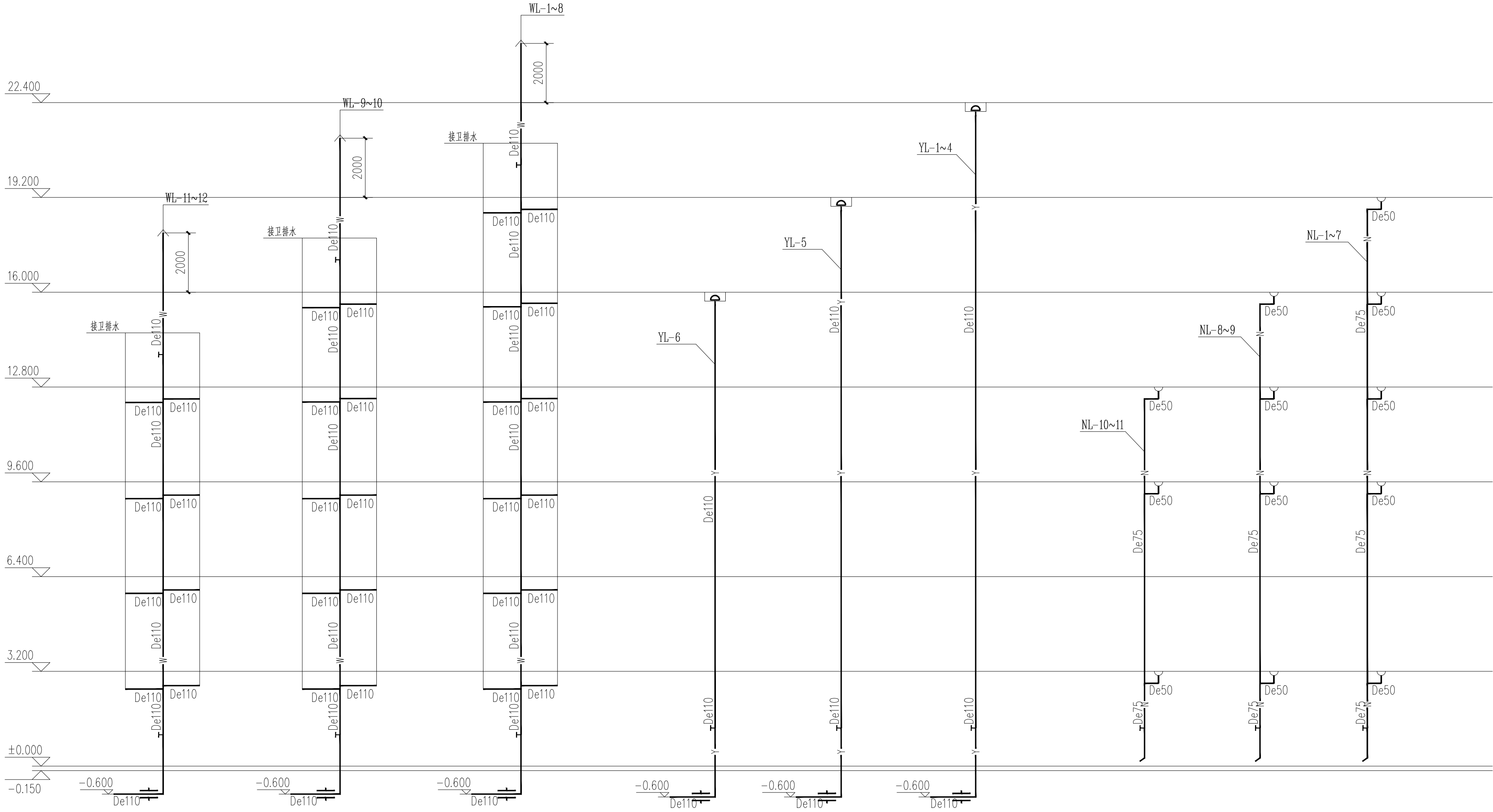
排水系统原理图
