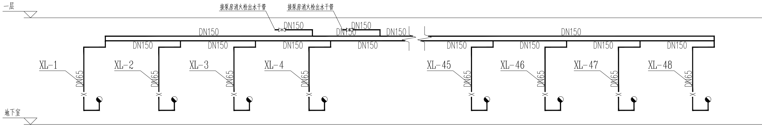
地下车库消火栓系统原理图
