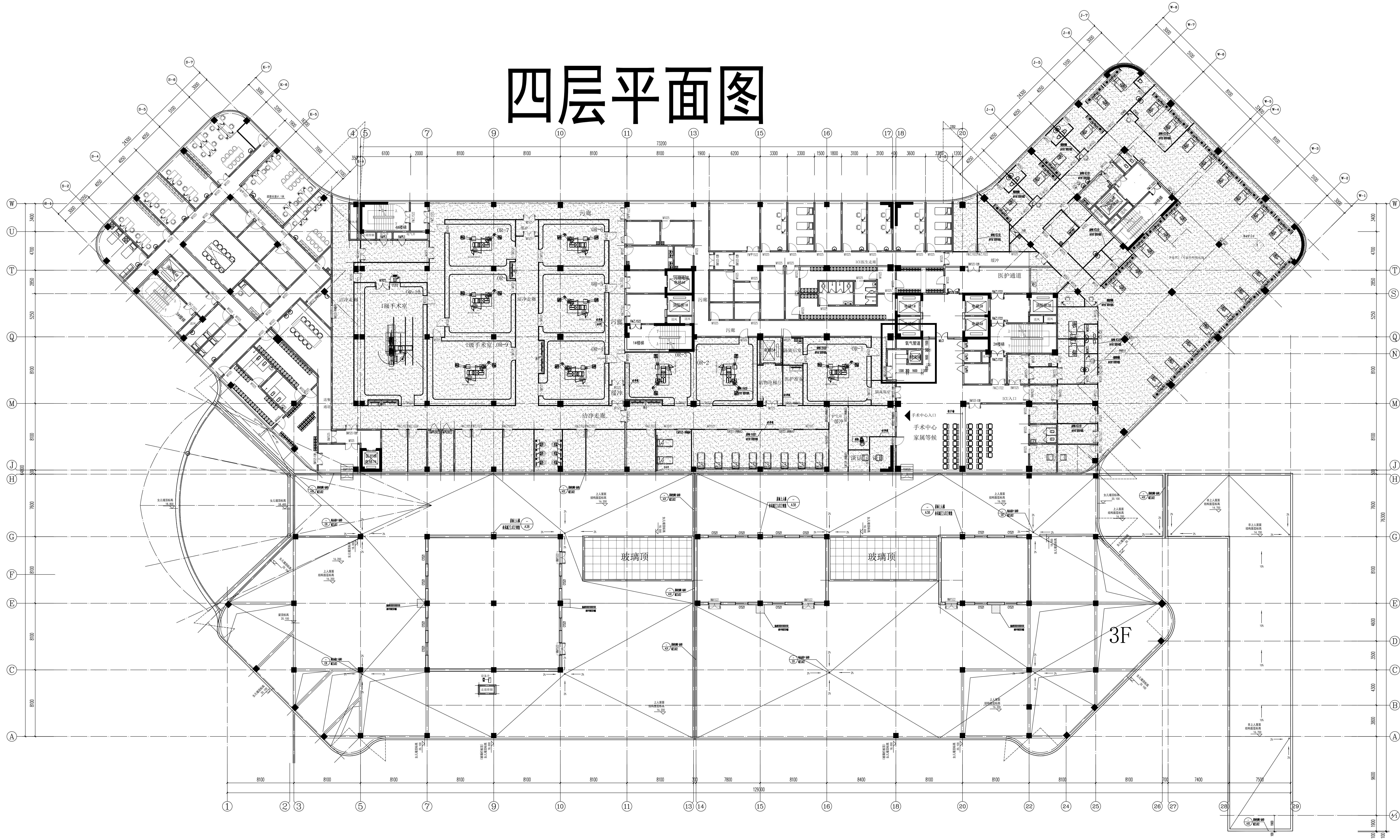
四层平面图 1:150
