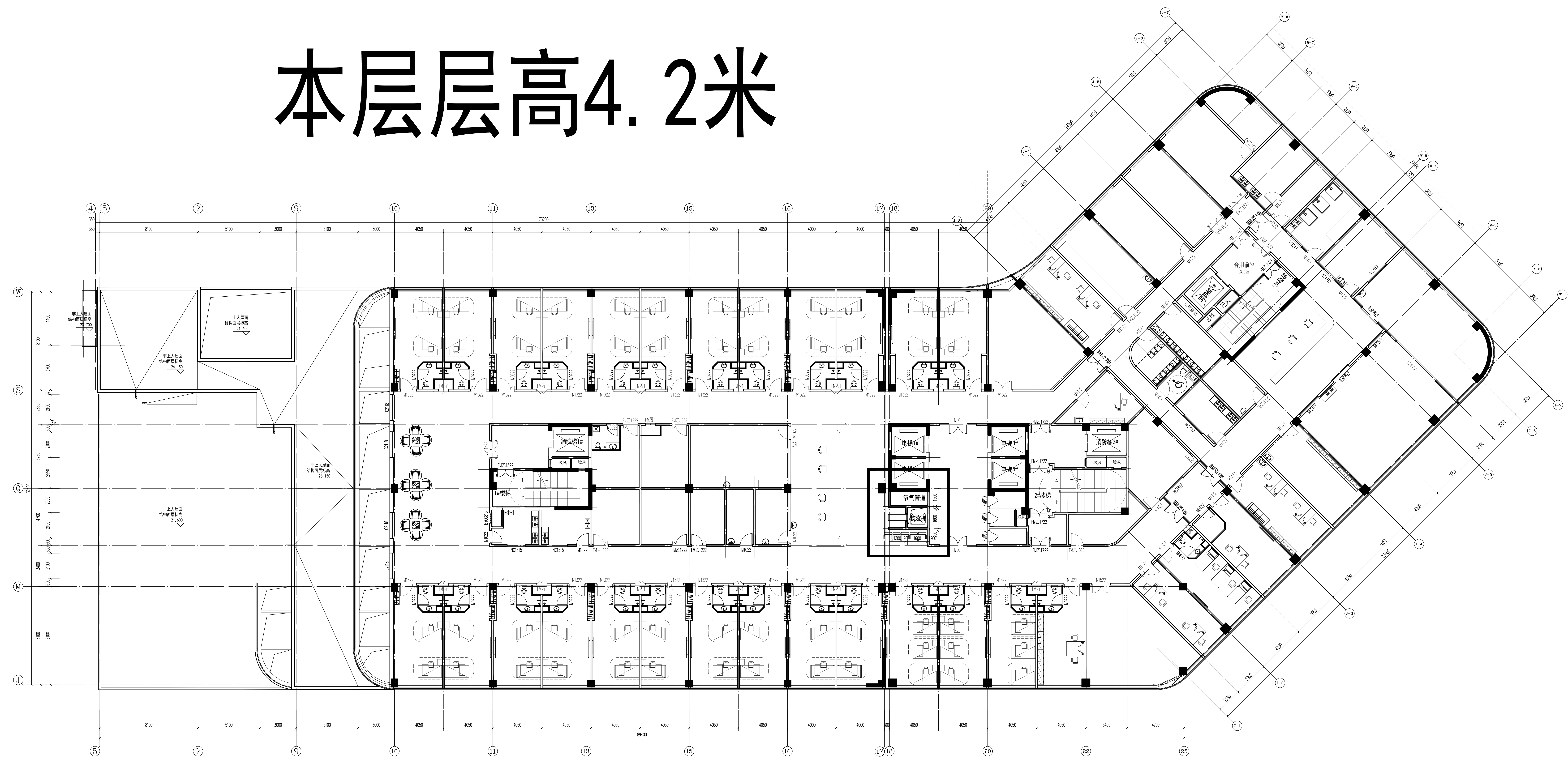
六层平面图 1:100
