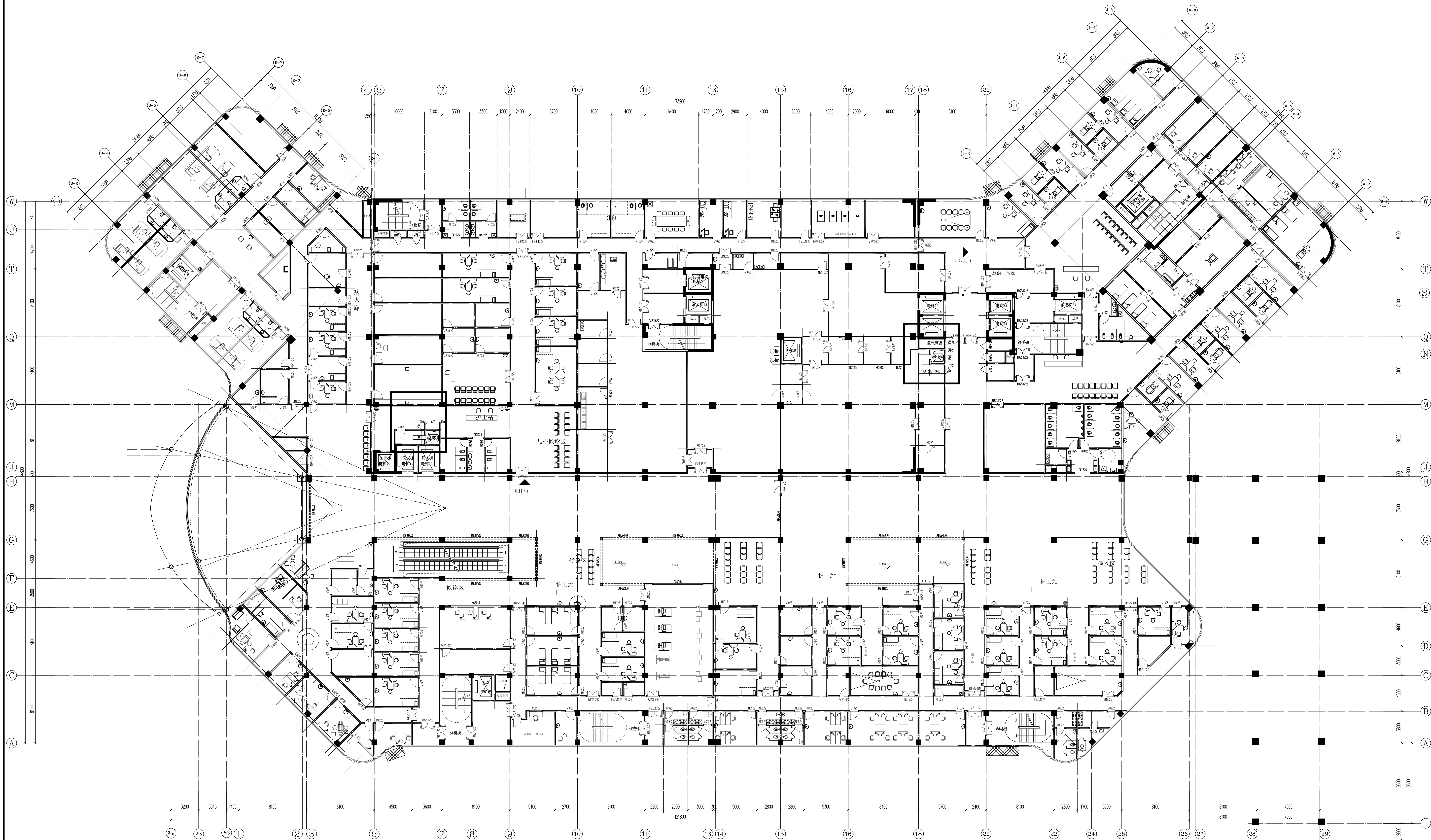
二层平面图 1:150
