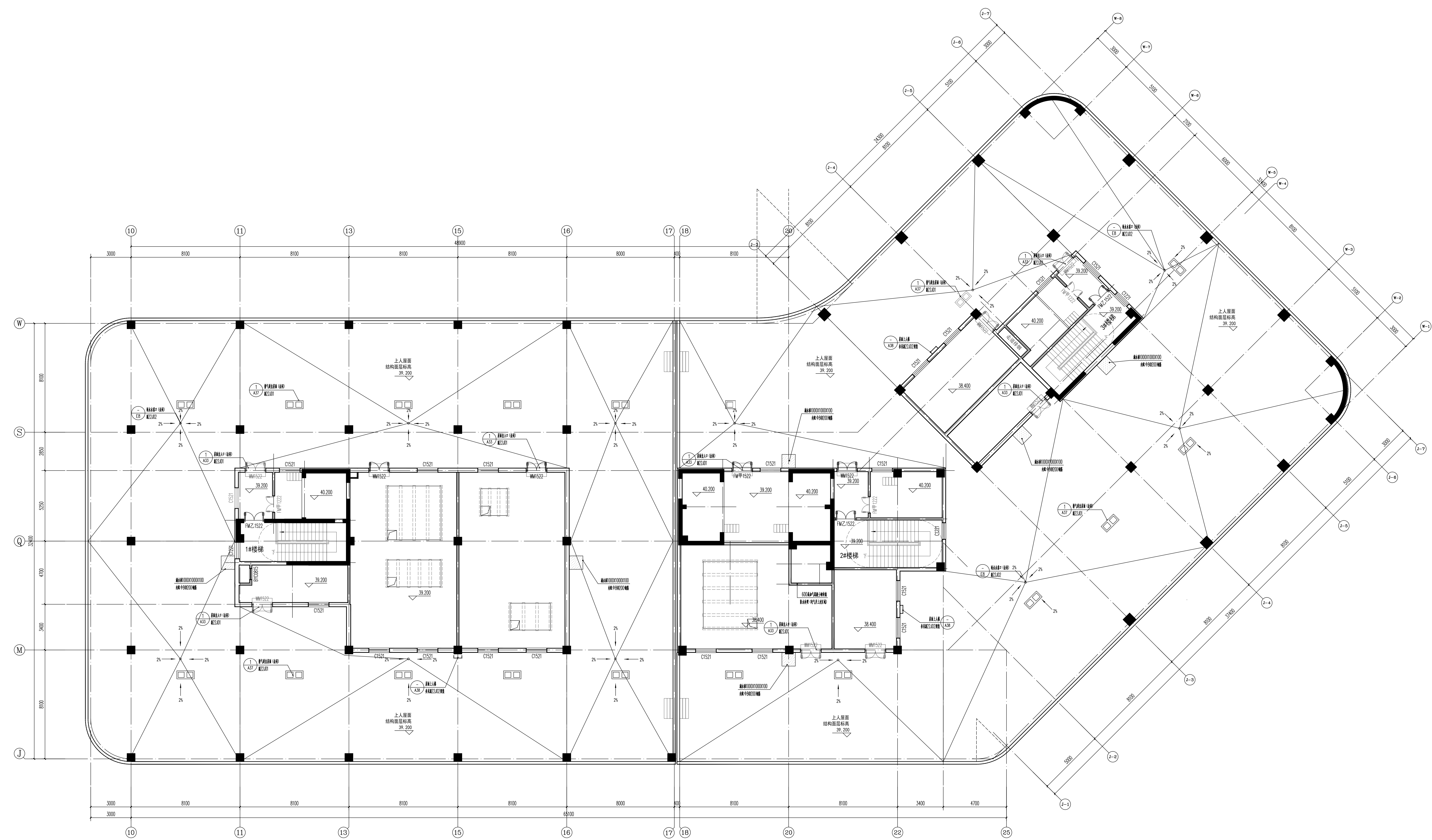
屋顶排水平面图 1:100
