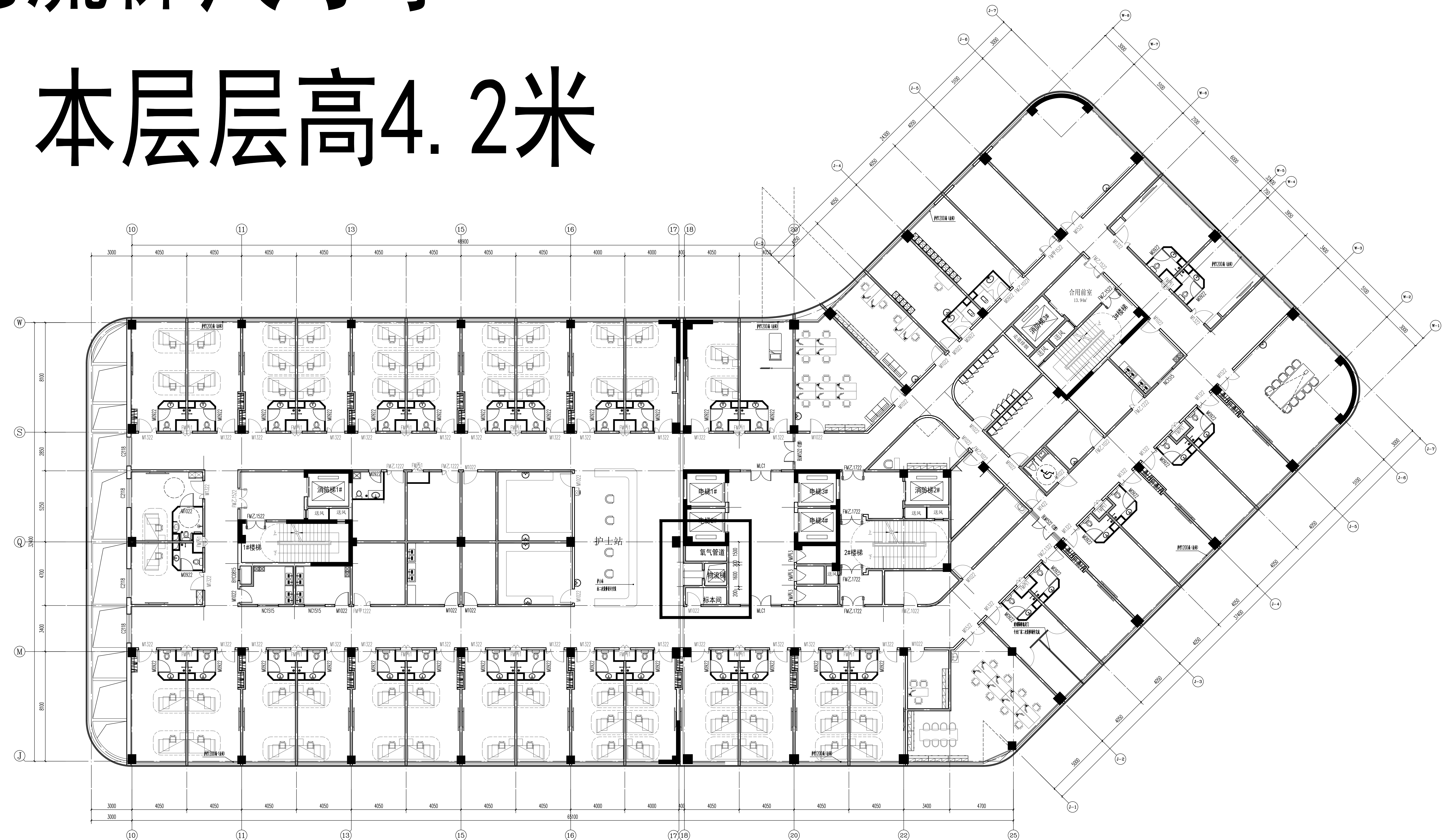
七层平面图 1:100
