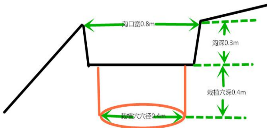
水平沟图示
