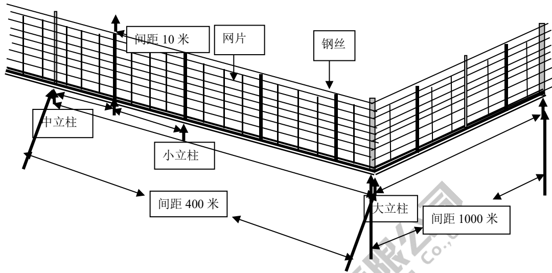
图 6-2-2 角铁网围栏安装示意图
