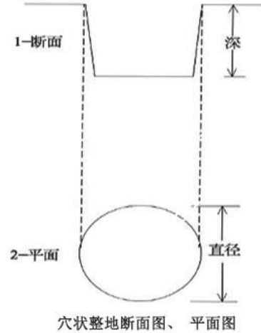
穴状整地断面图、平面图
