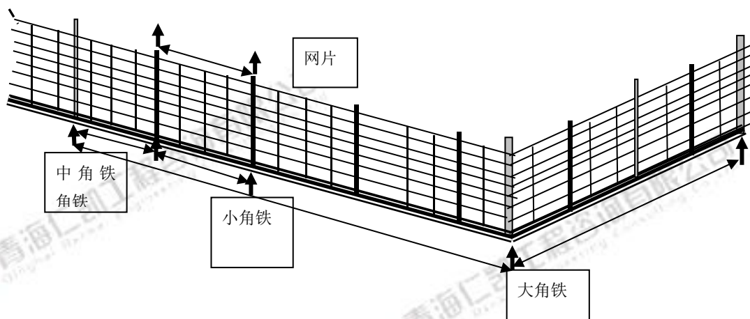
图6-1 角铁网围栏安装示意图
