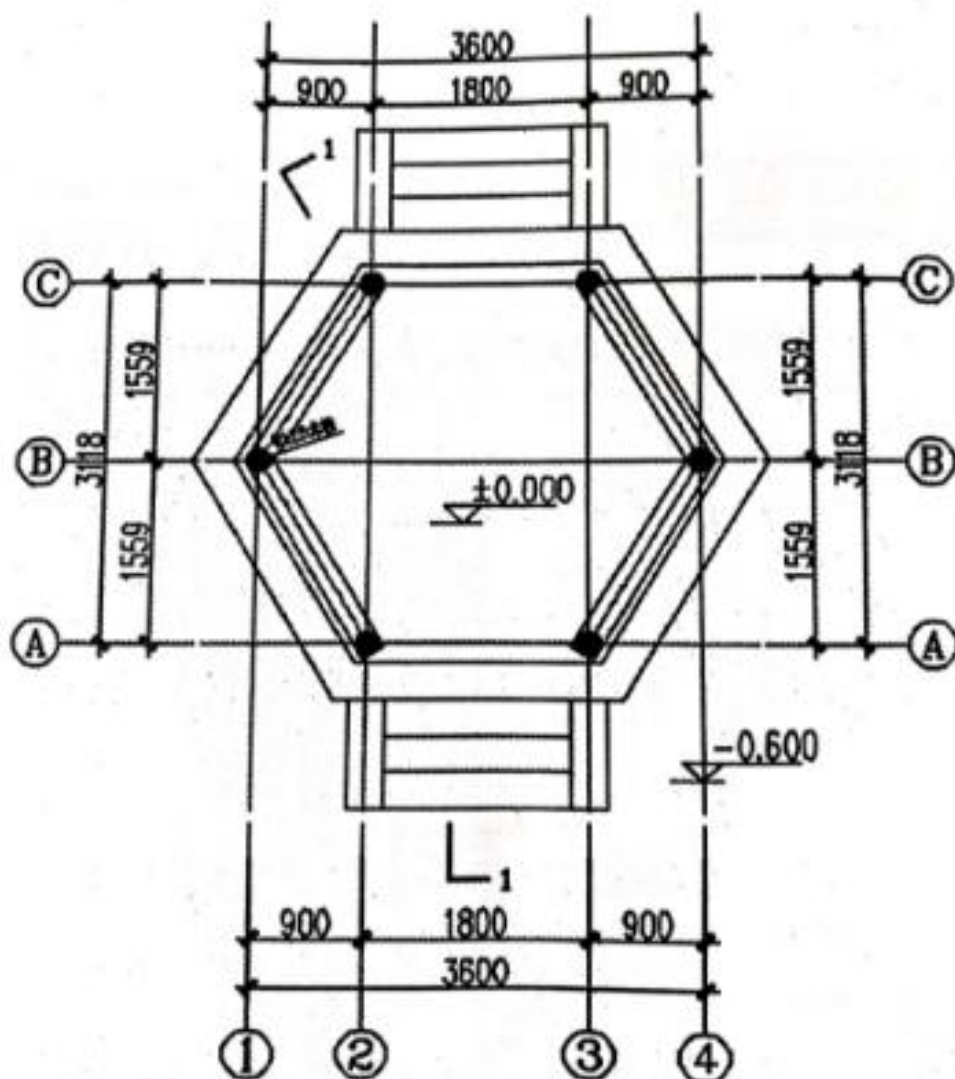
六角亭平面图
