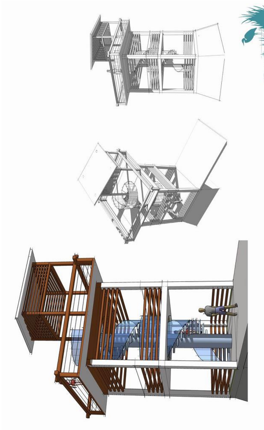
观景台透视图
