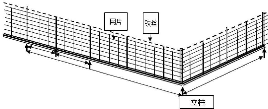
网围栏安装示意图
