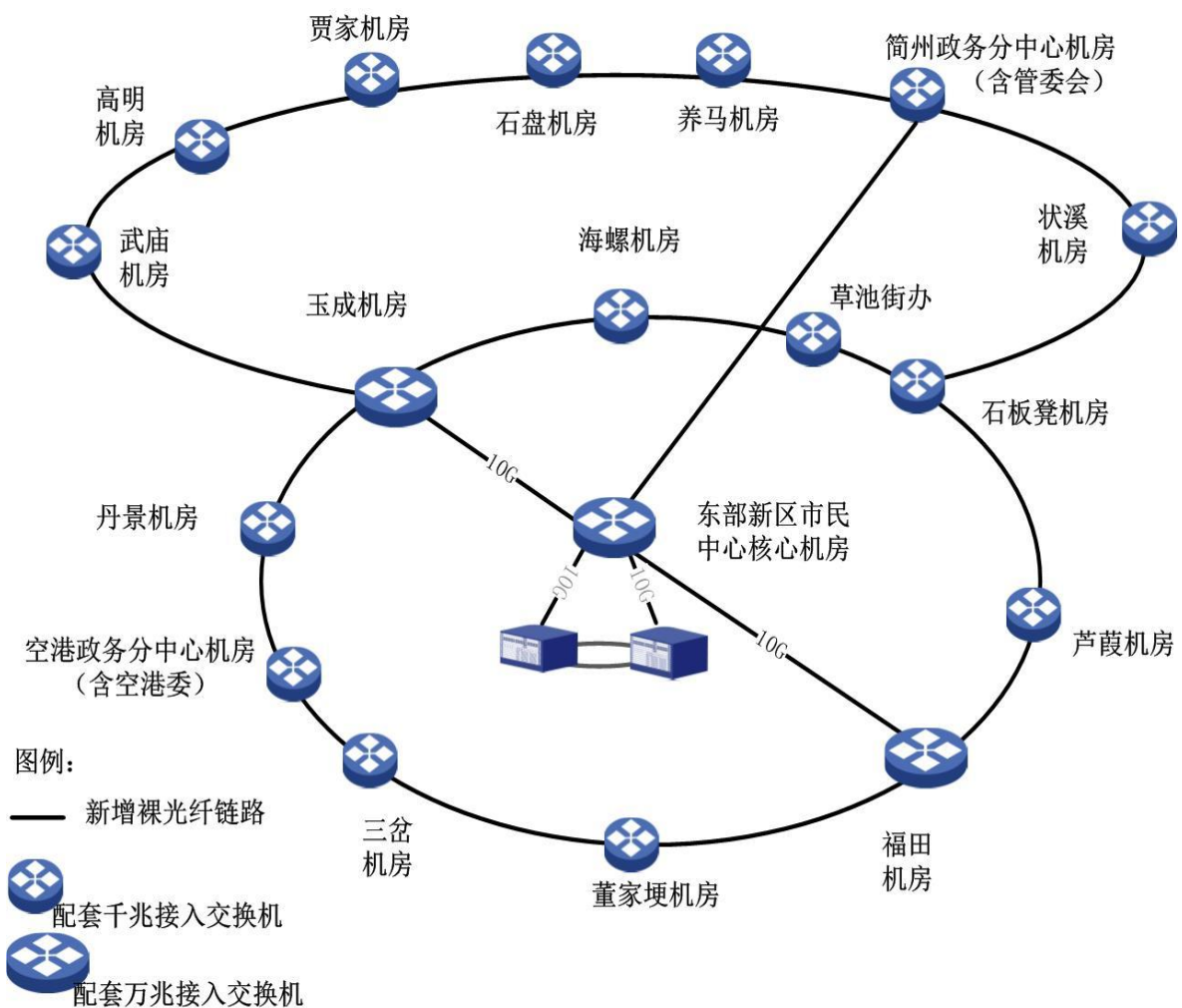
成都市东部新区电子政务外网接入网络及光纤路由图
